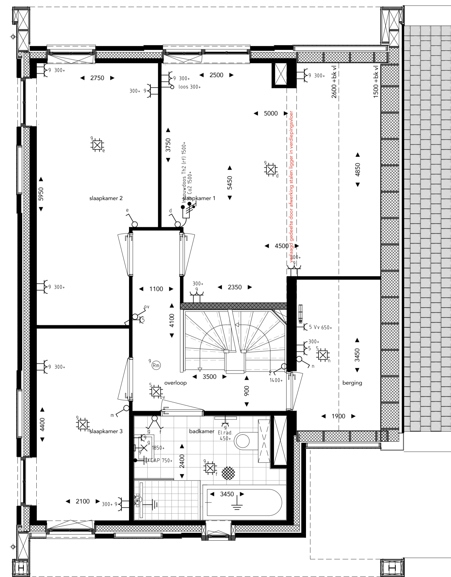
eerste verdieping
