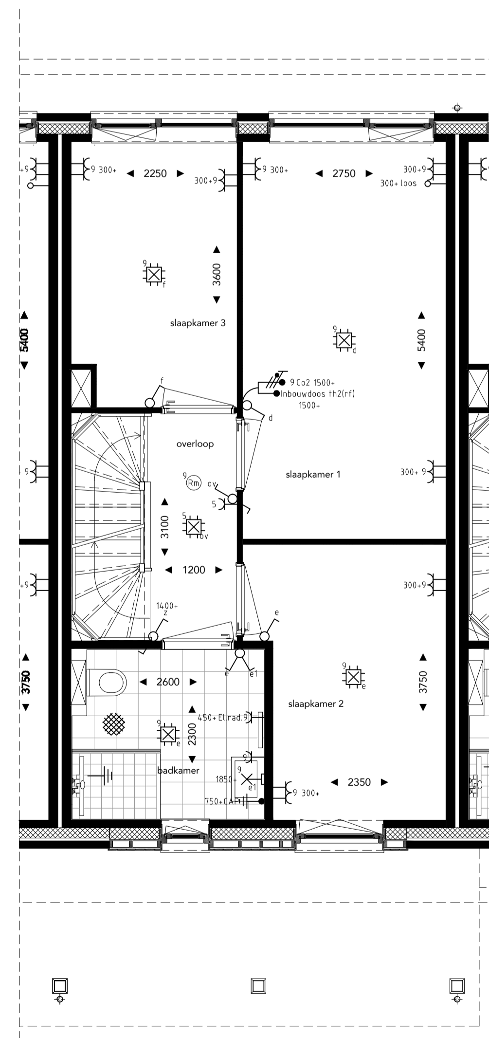
eerste verdieping
