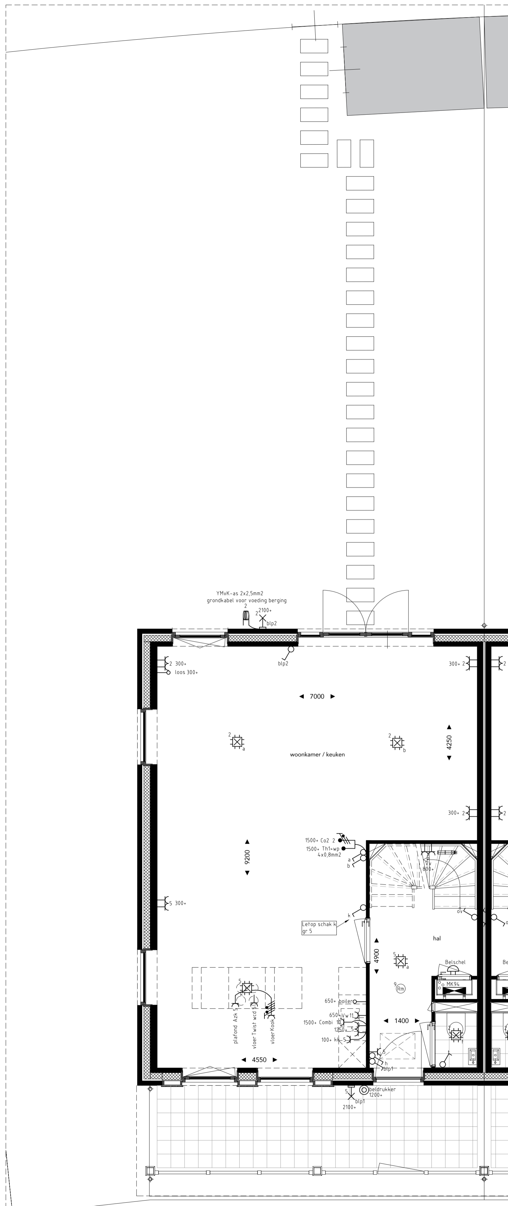
begane grond
