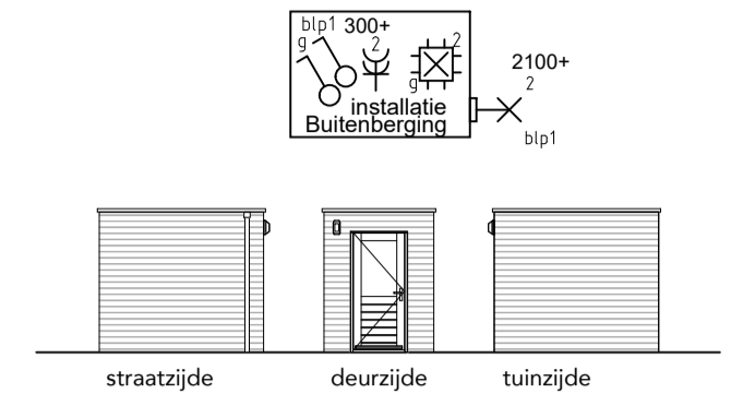
schuur schaal 1 : 150
