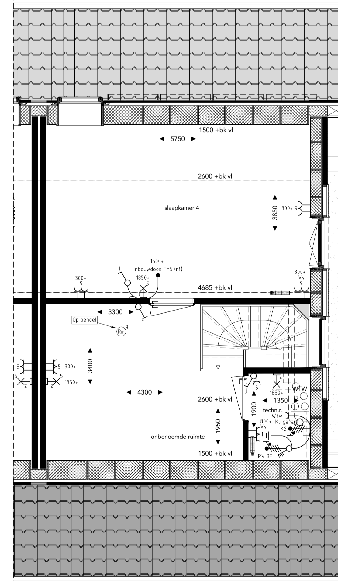
tweede verdieping
