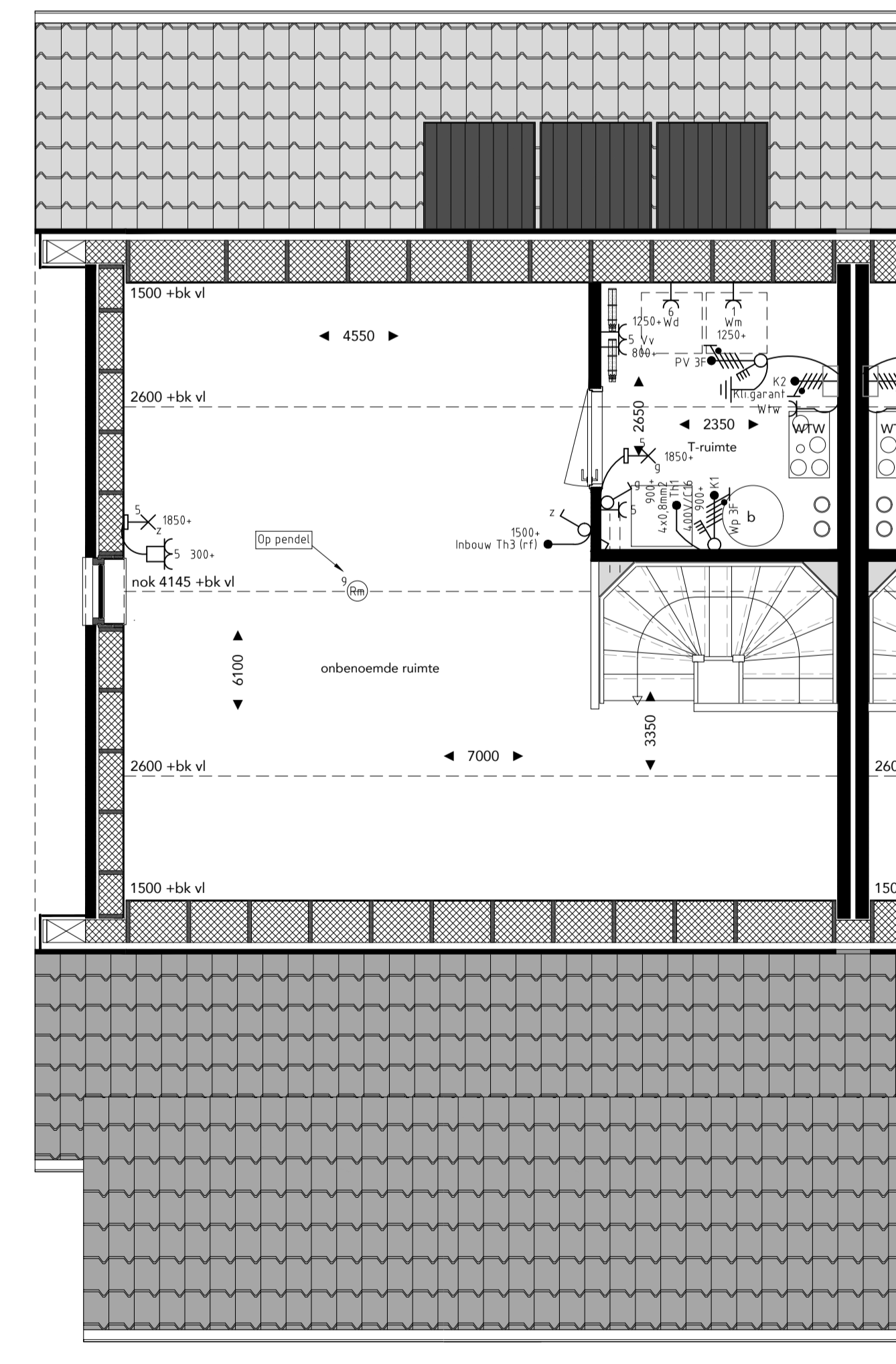
tweede verdieping
