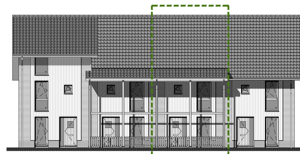
voorgevel schaal 1 : 150
