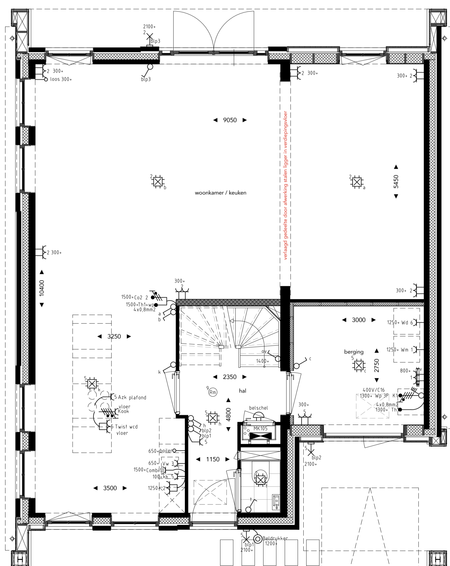
begane grond
