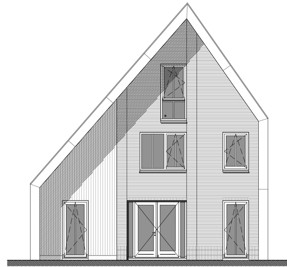
achtergevel schaal 1 : 100
