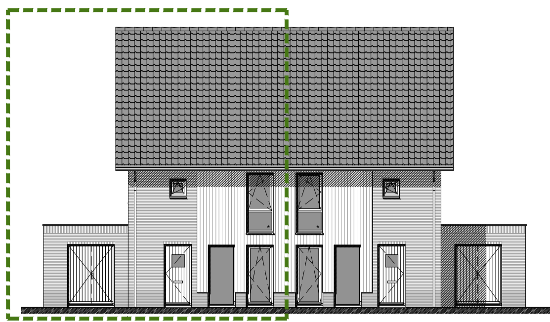
voorgevel schaal 1 : 150
