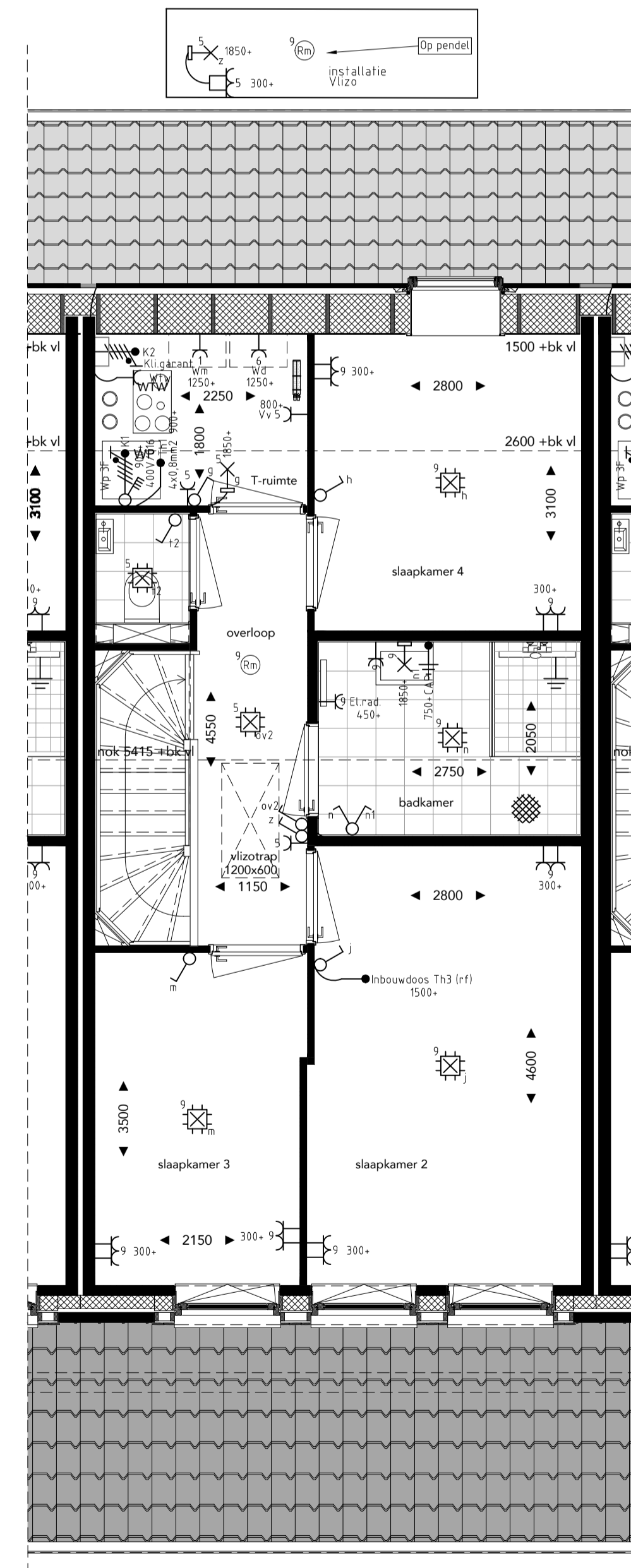
tweede verdieping
