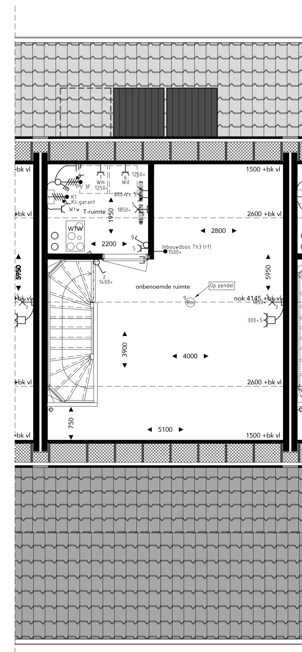
tweede verdieping
