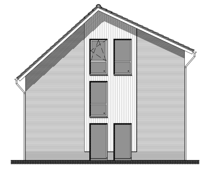
zijgevel schaal 1 : 150
