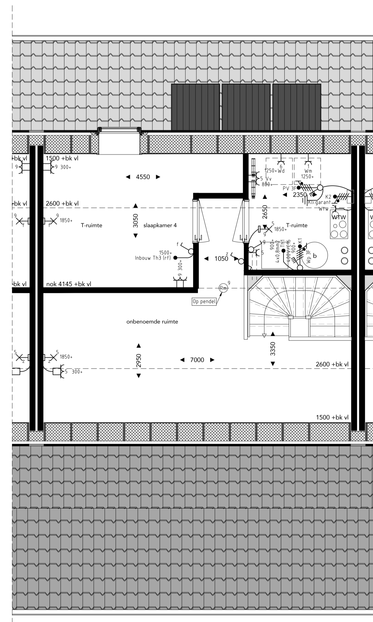
tweede verdieping
