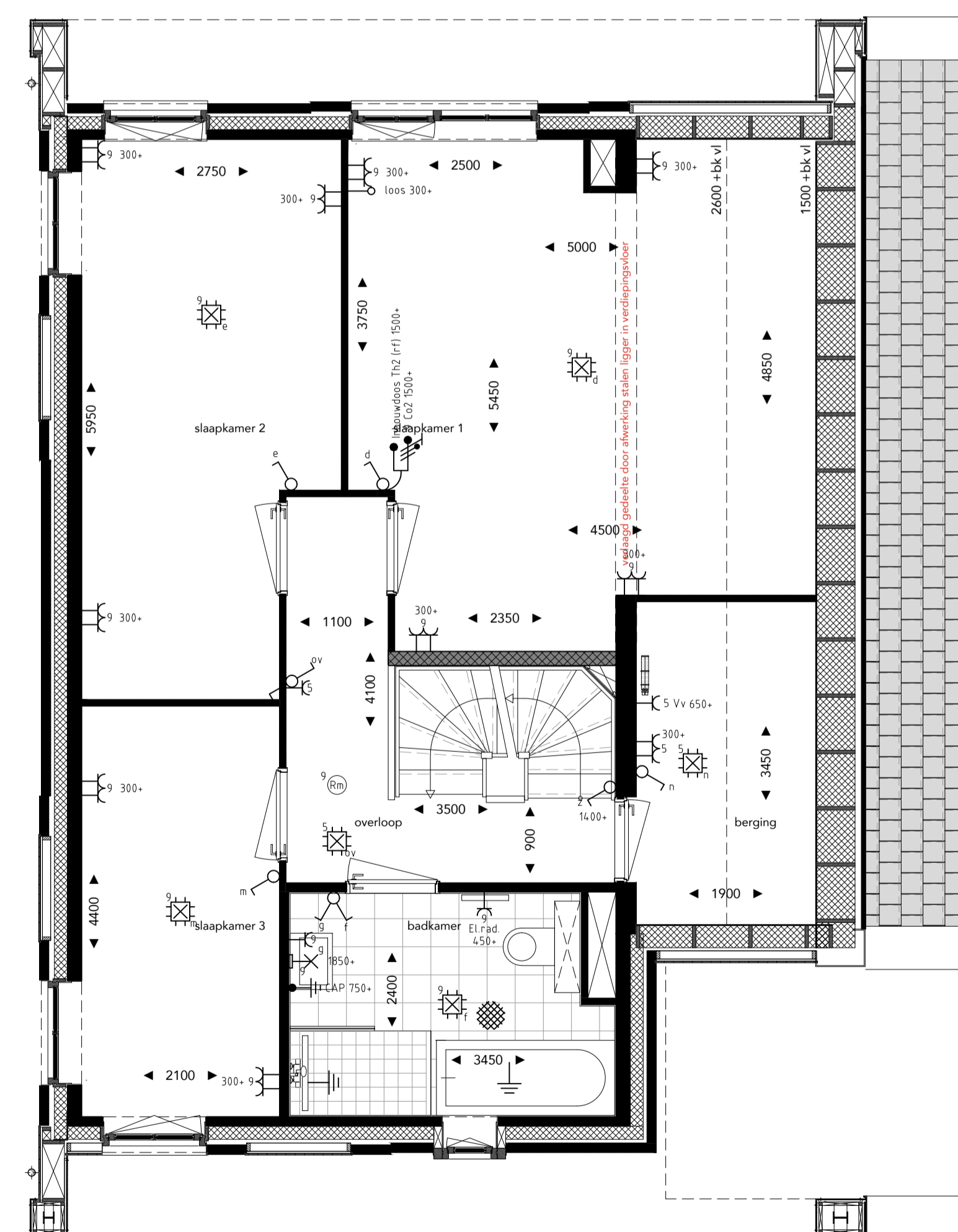
eerste verdieping
