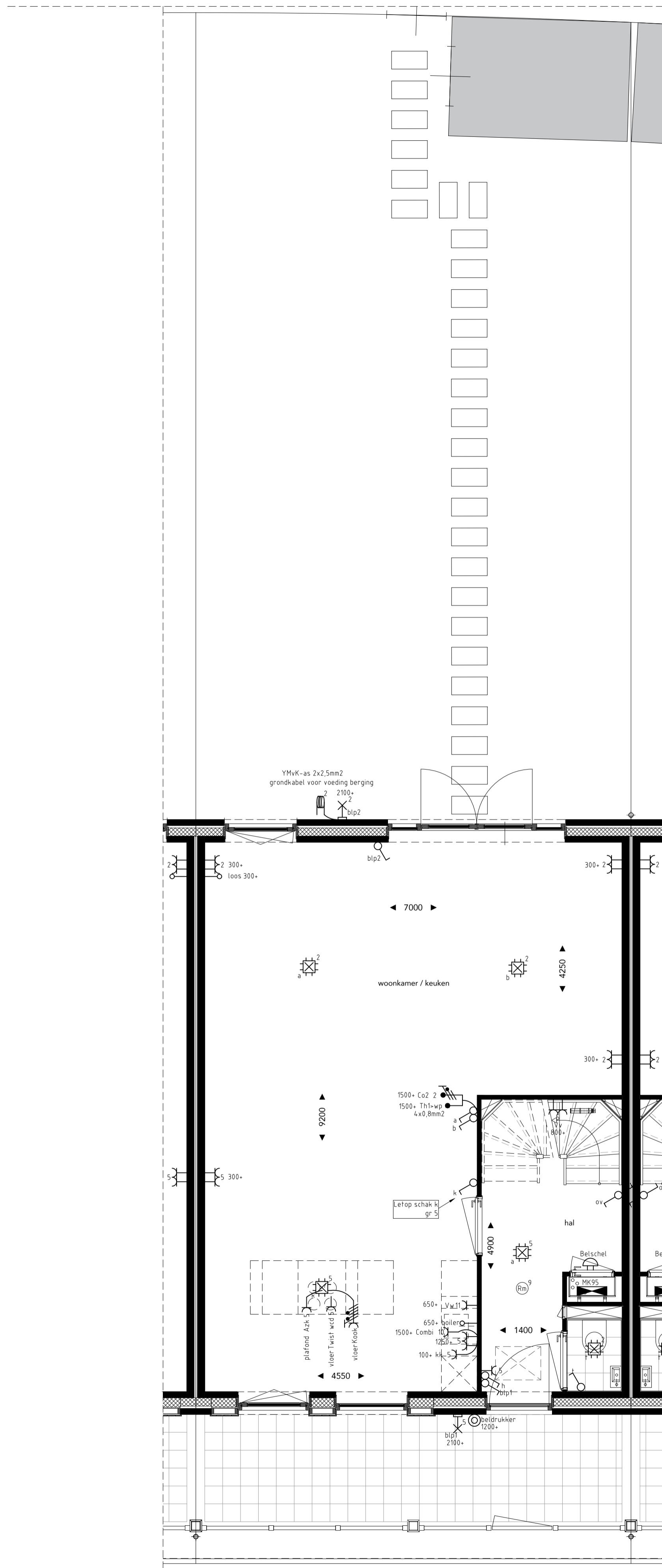
begane grond
