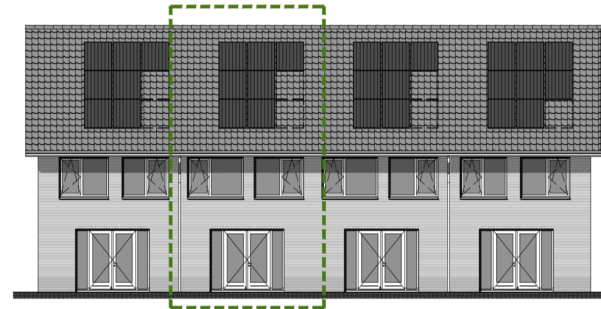
achtergevel schaal 1 : 150
