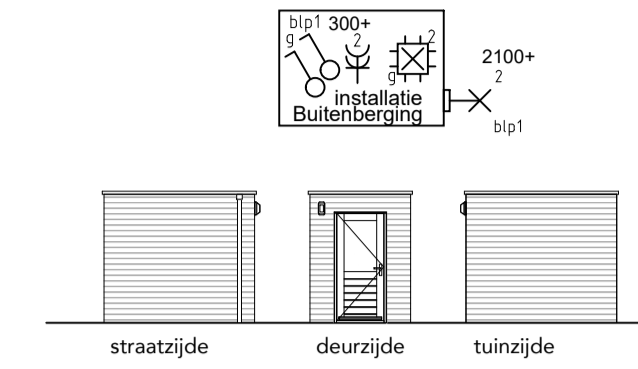
schuur schaal 1 : 150
