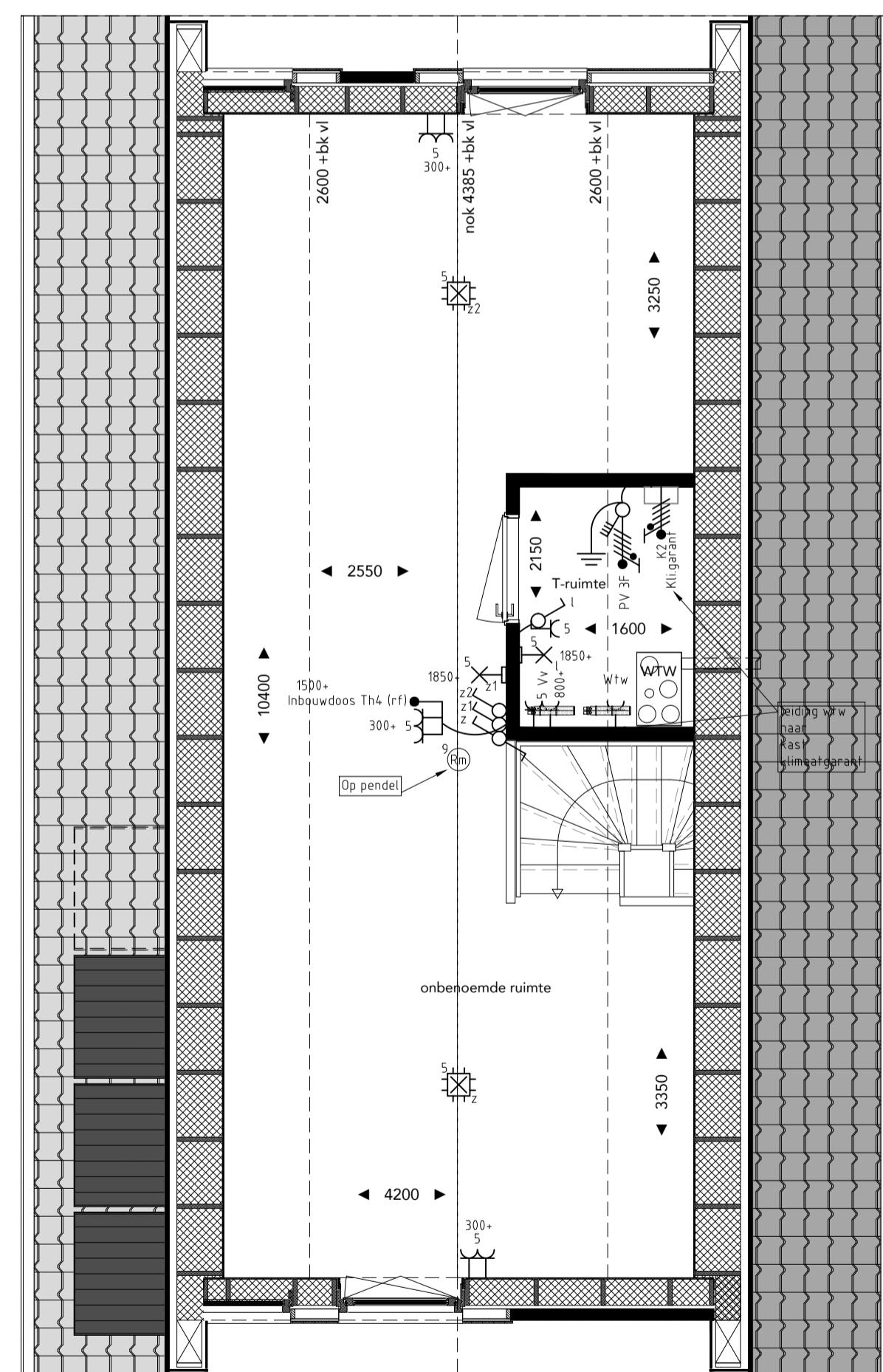
tweede verdieping
