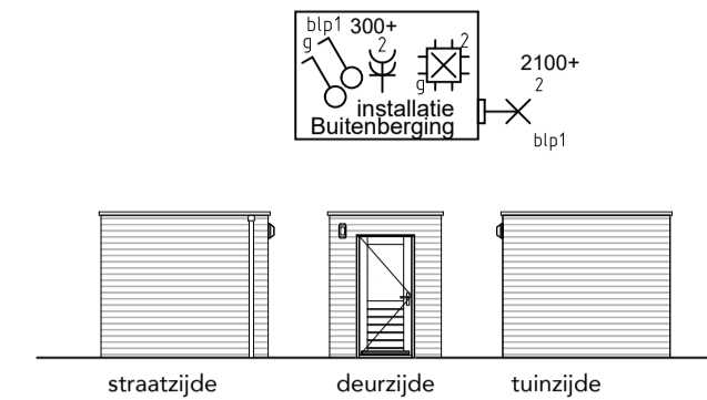
schuur schaal 1 : 150
