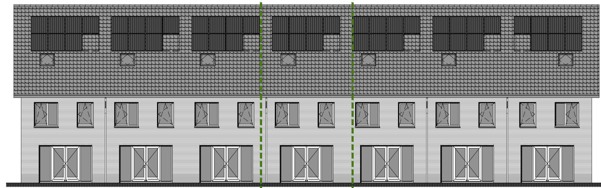
achtergevel schaal 1 : 150
