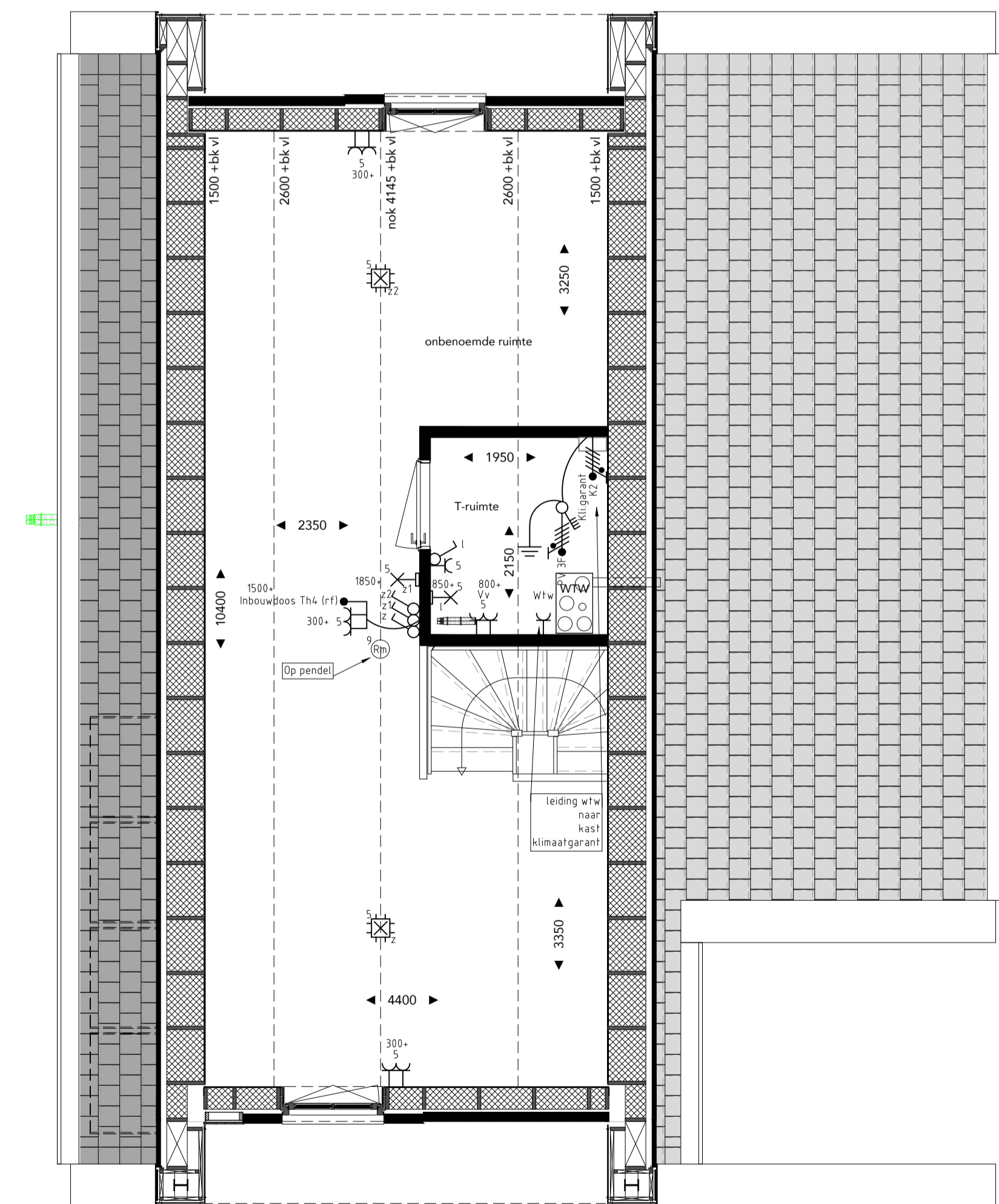
tweede verdieping
