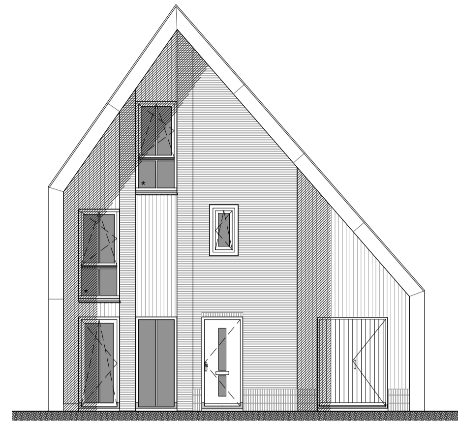
voorgevel schaal 1 : 100
