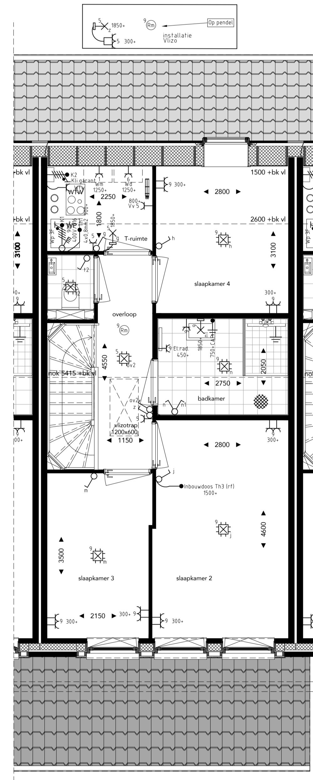
tweede verdieping
