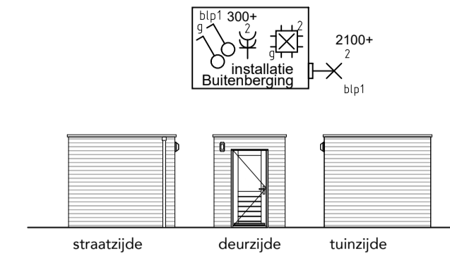
schuur schaal 1 : 150
