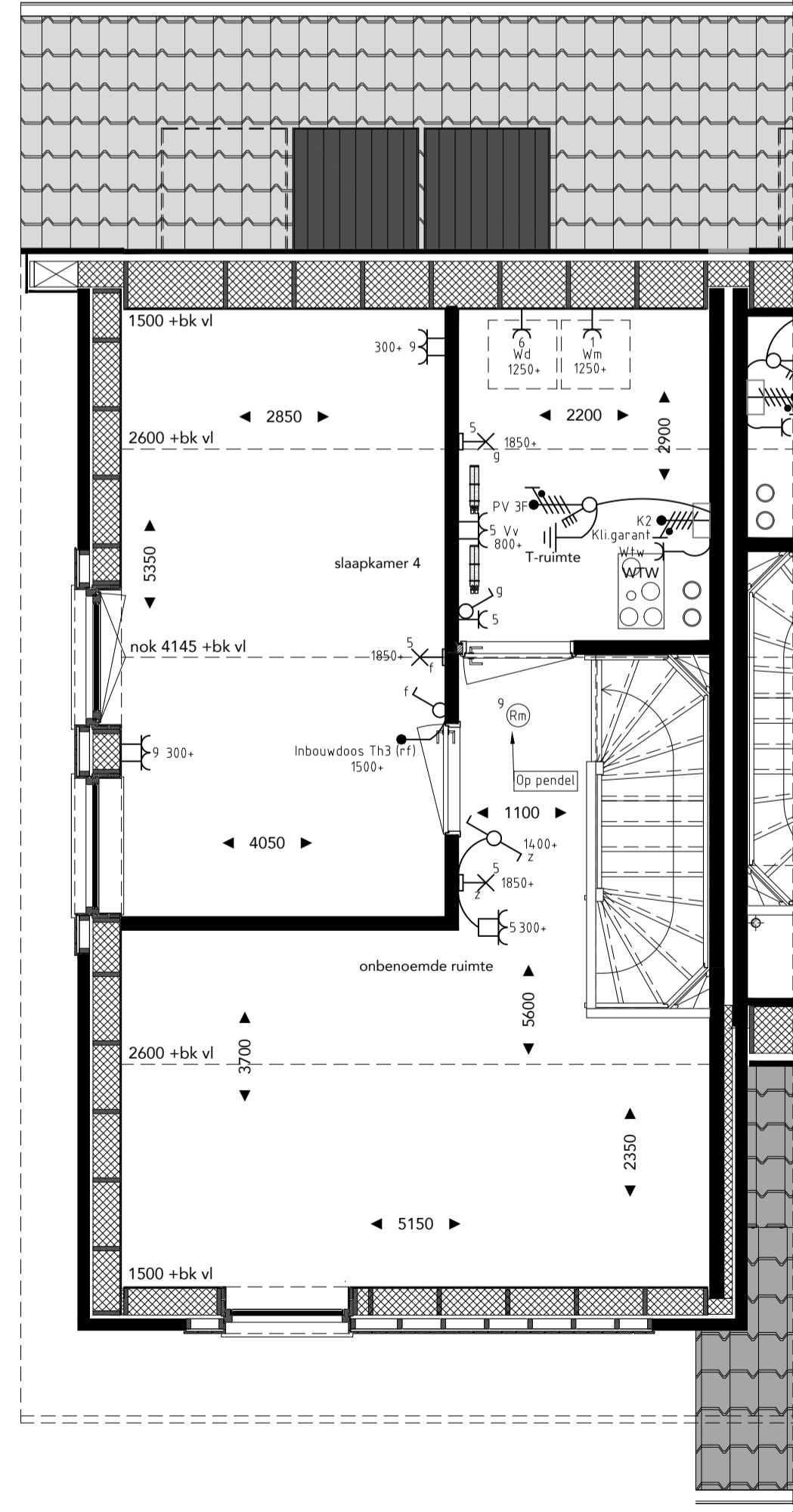
tweede verdieping
