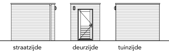
schuur schaal 1 : 150
