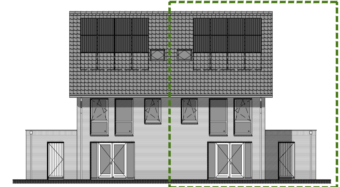
achtergevel schaal 1 : 150
