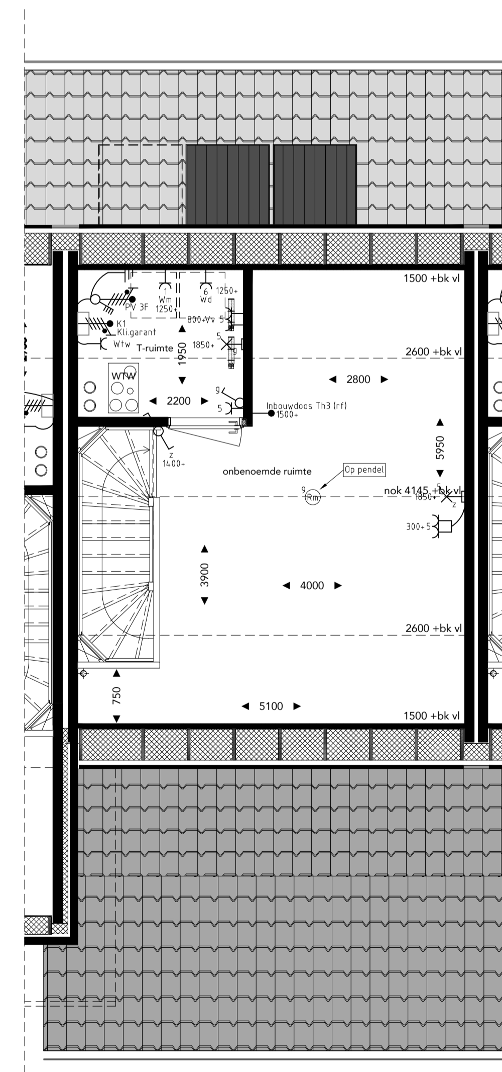
tweede verdieping
