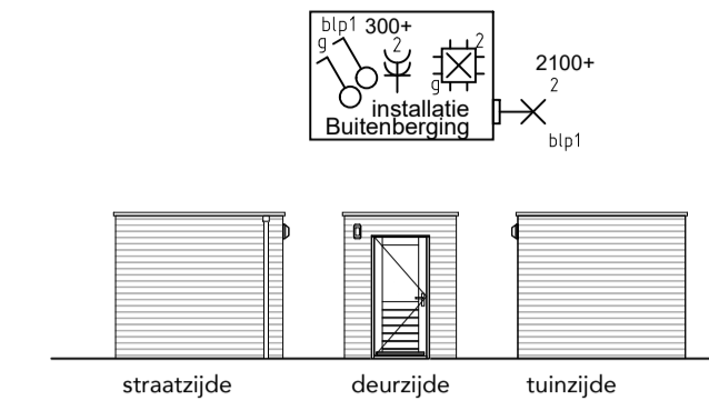
schuur schaal 1 : 150
