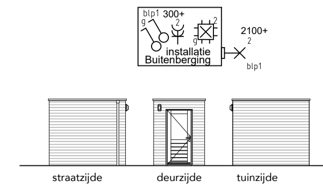
schuur schaal 1 : 150
