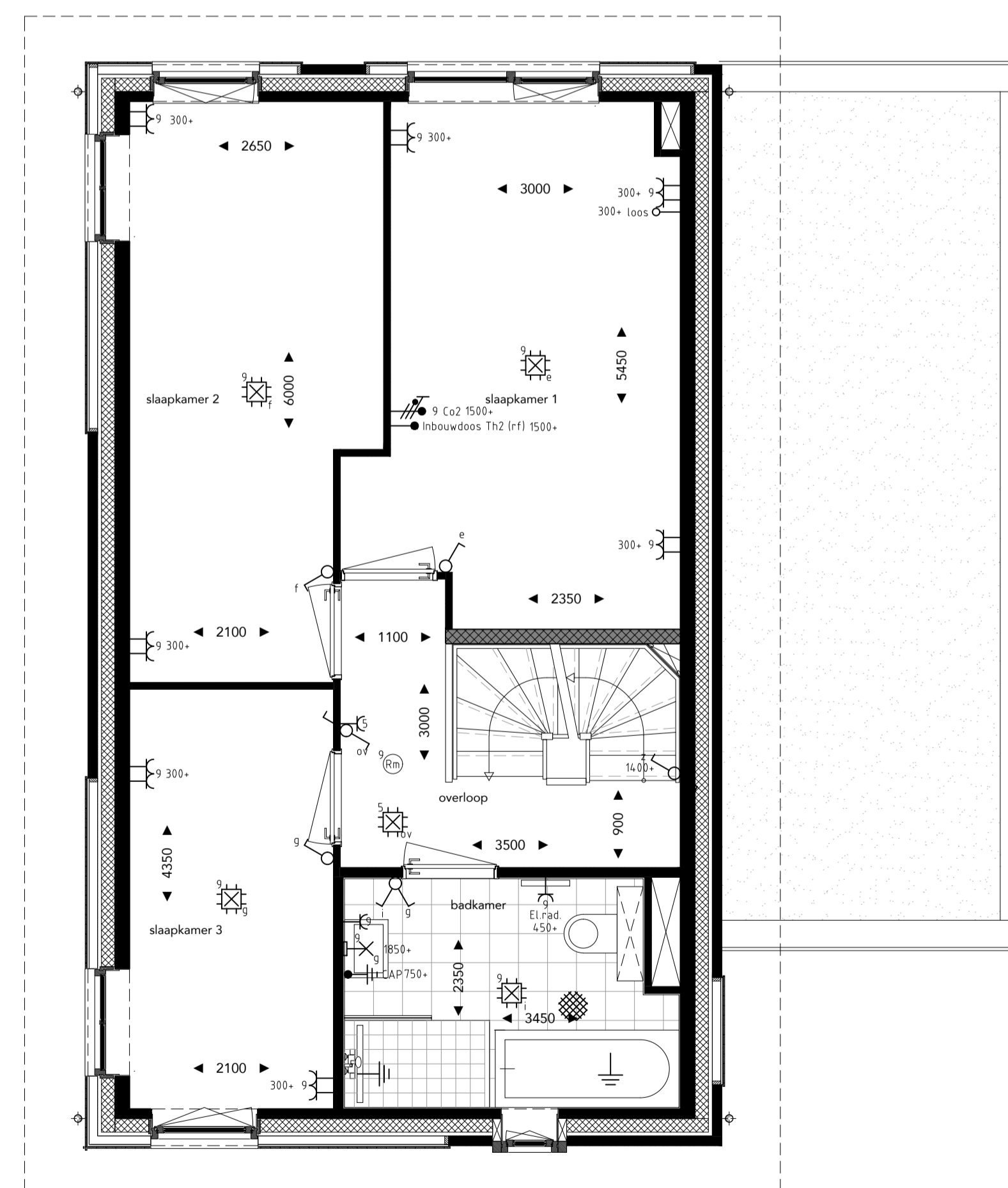
eerste verdieping
