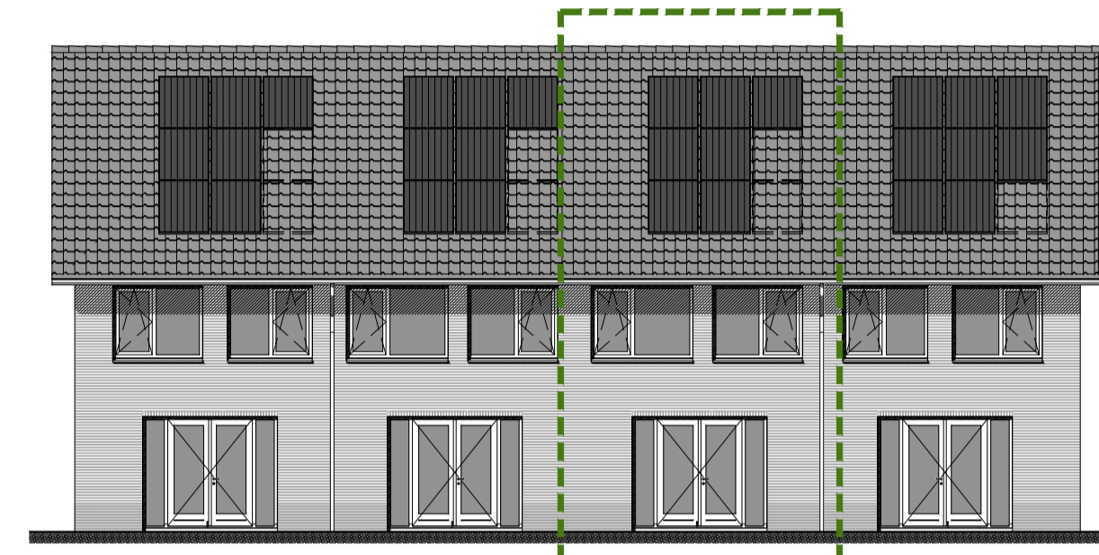
achtergevel schaal 1 : 150
