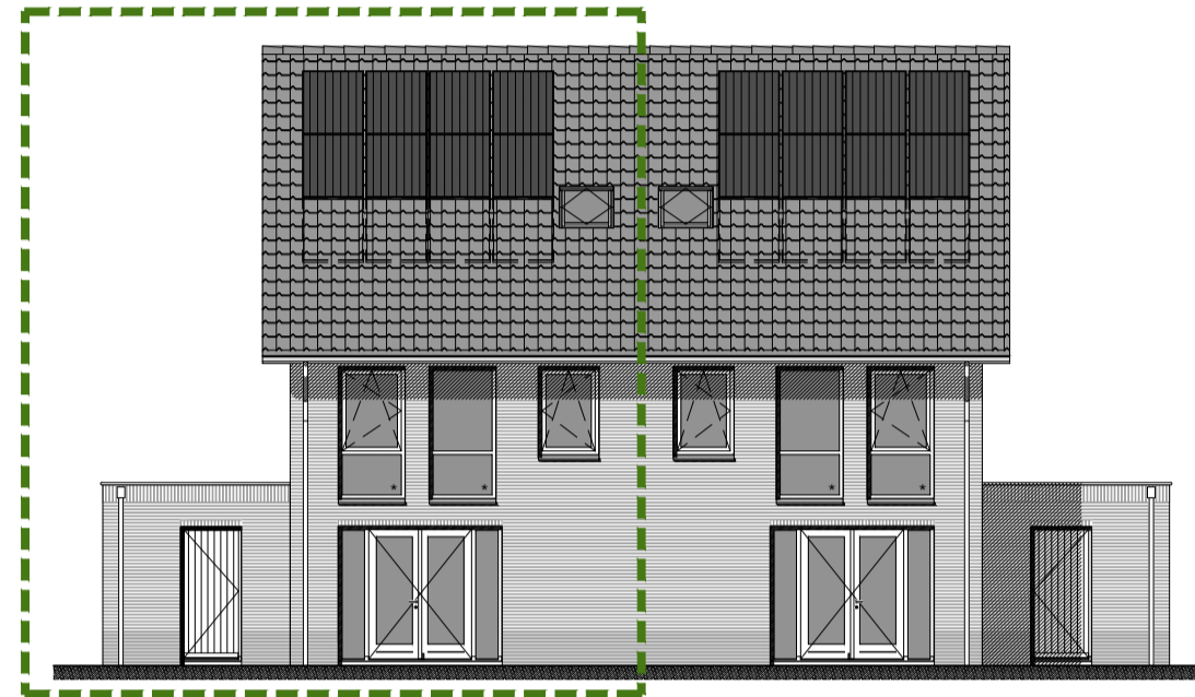
achtergevel schaal 1 : 150
