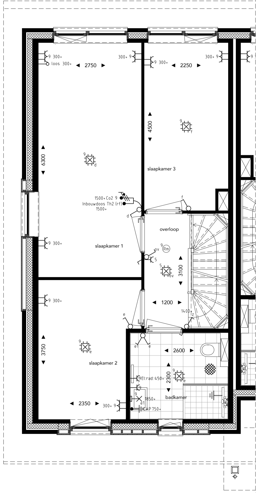
eerste verdieping
