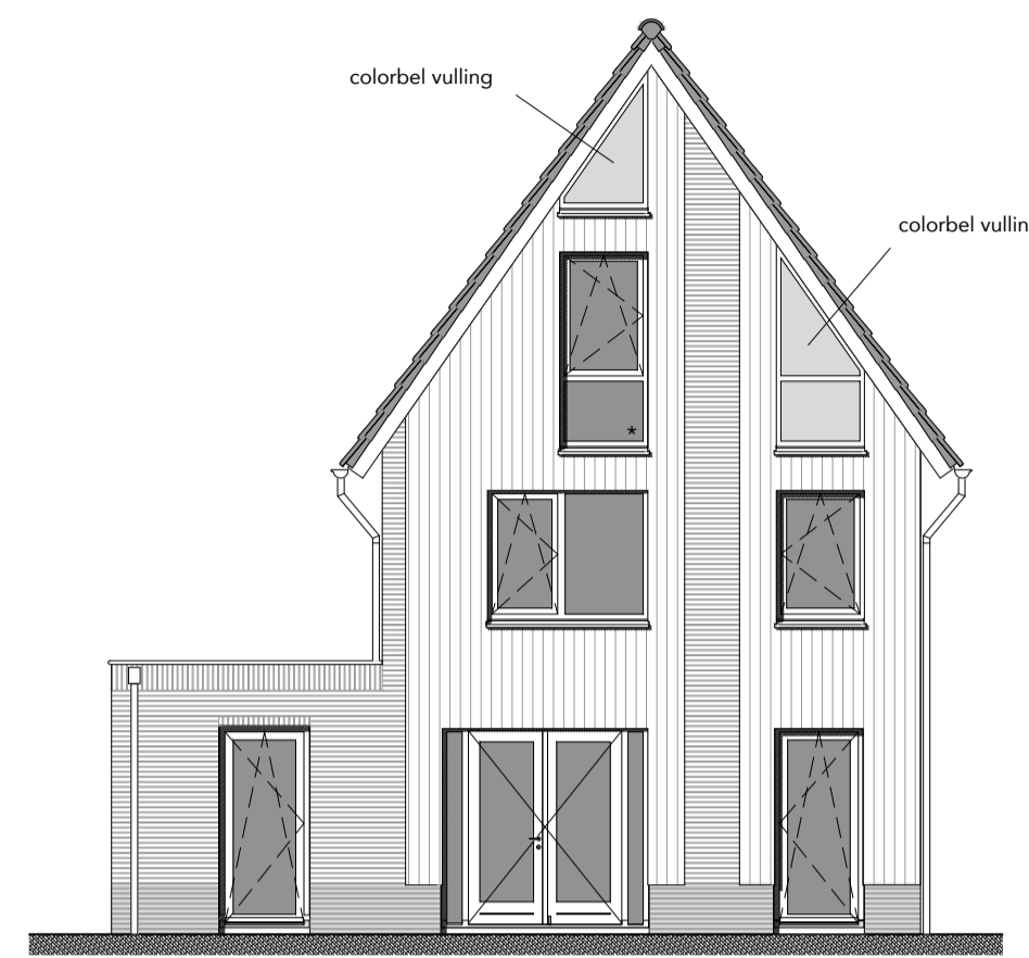
achtergevel schaal 1 : 100
