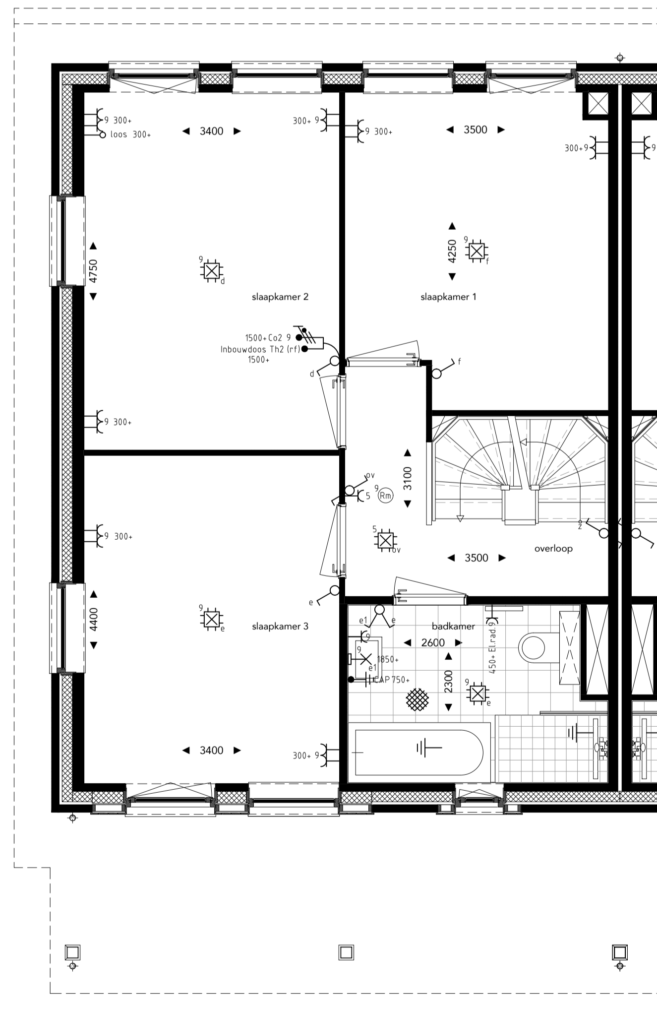
eerste verdieping
