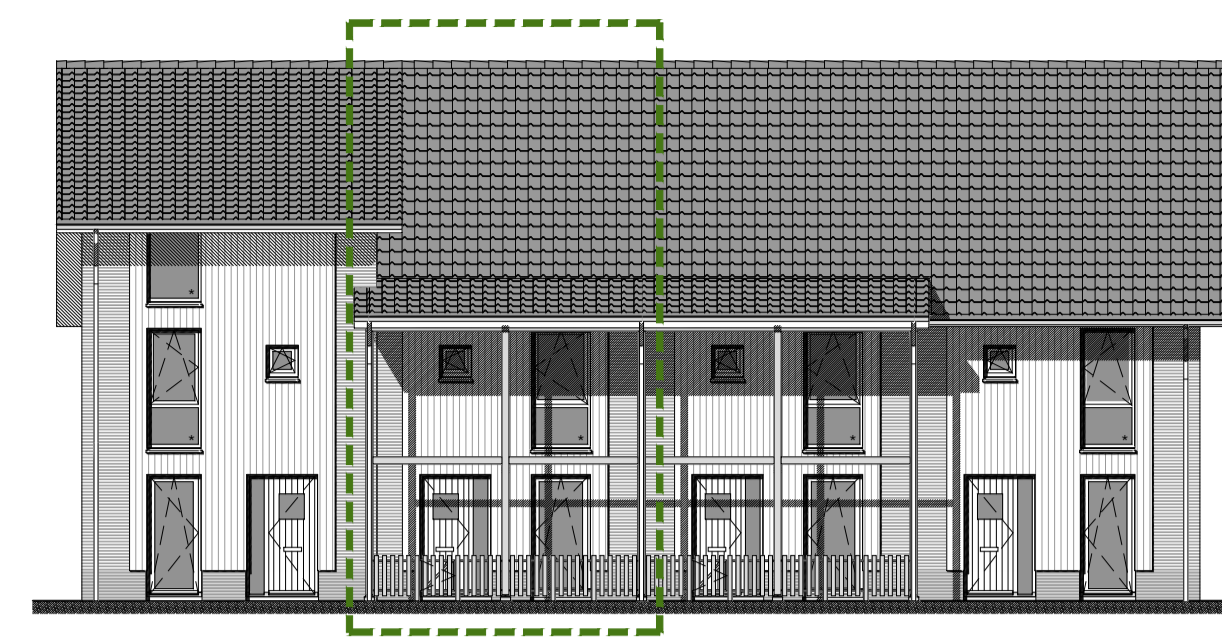
voorgevel schaal 1 : 150
