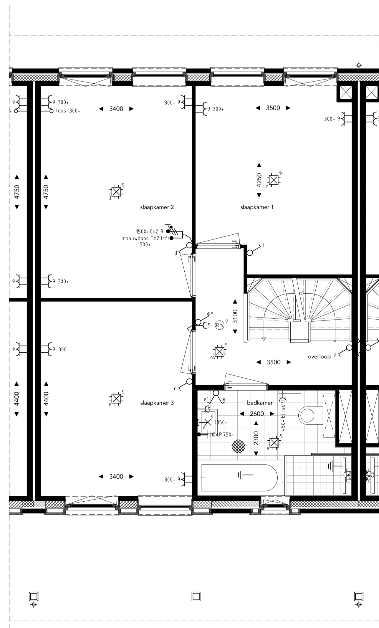
eerste verdieping
