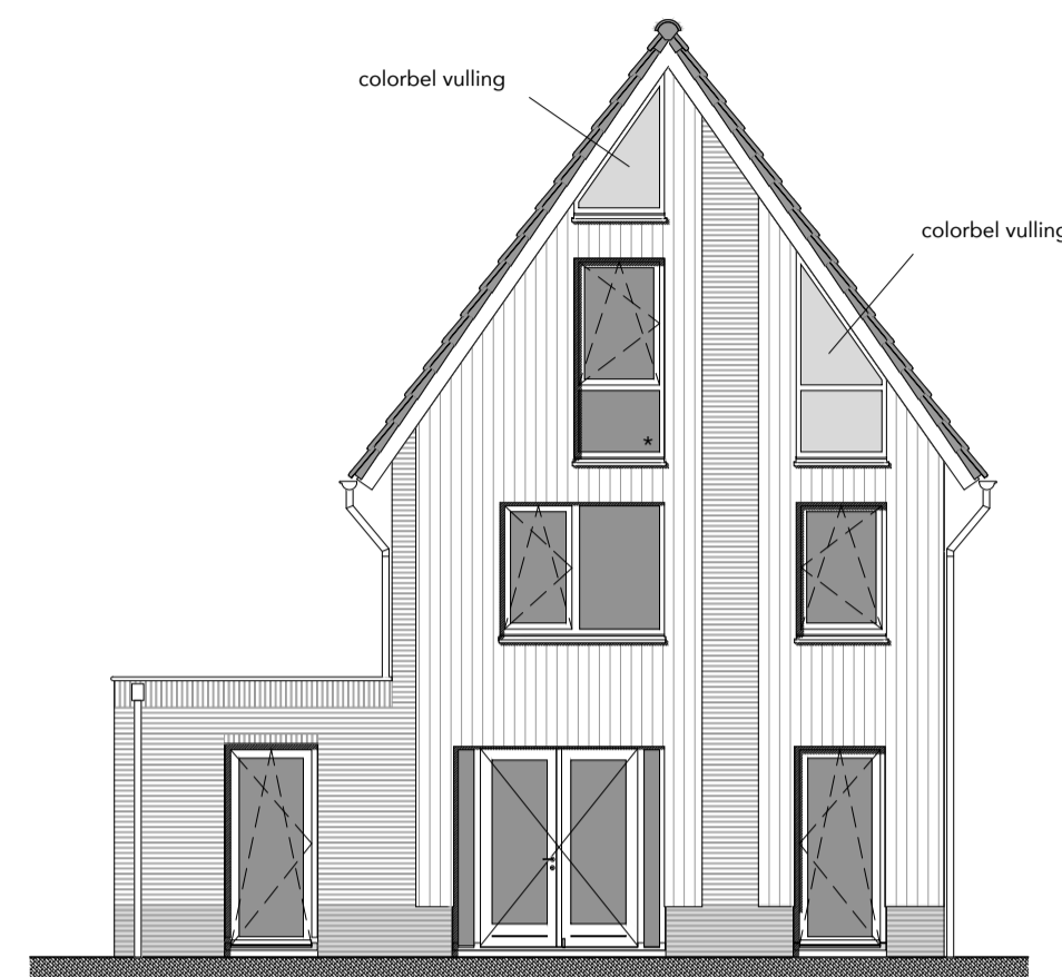
achtergevel schaal 1 : 100
