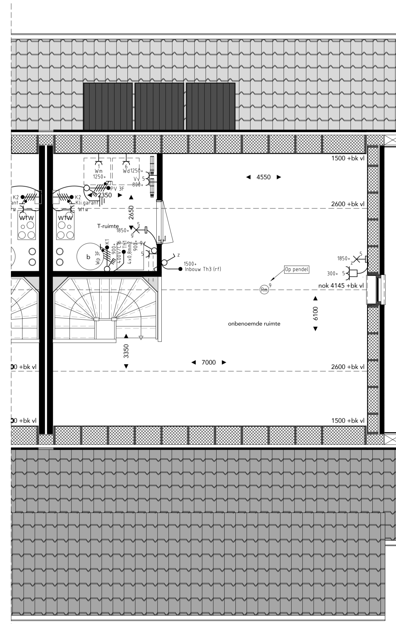
tweede verdieping
