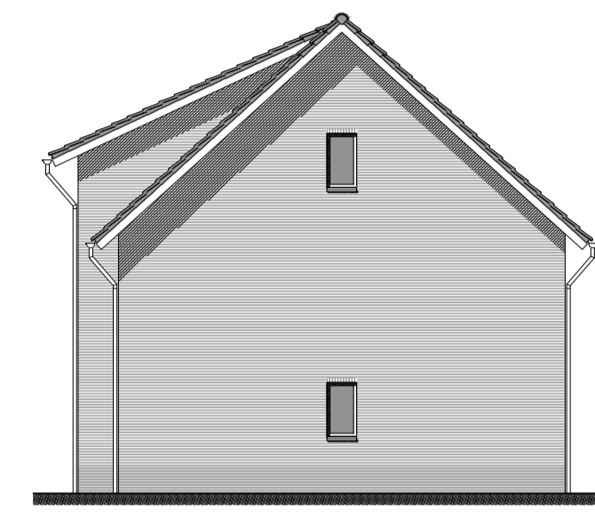
zijgevel schaal 1 : 150
