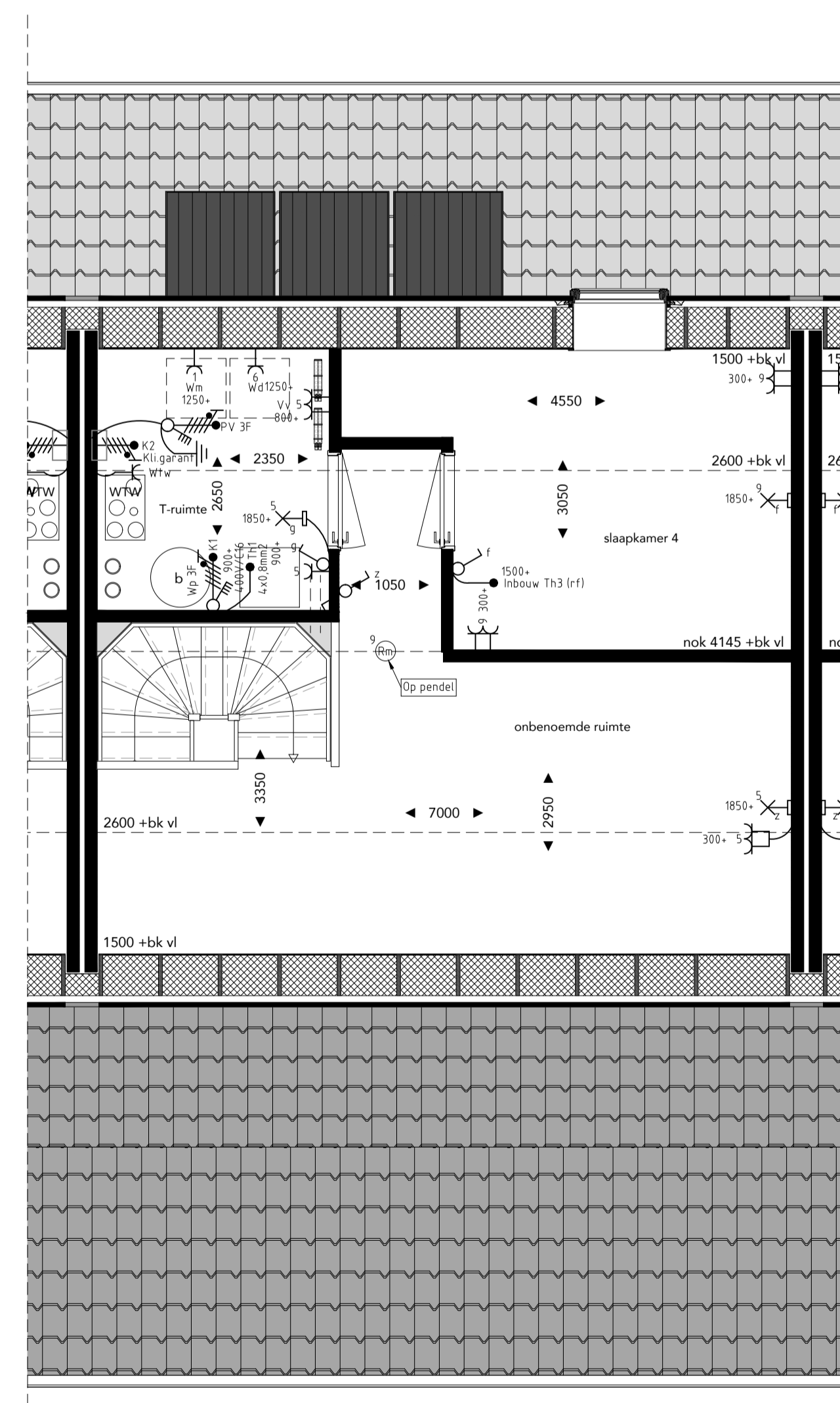
tweede verdieping
