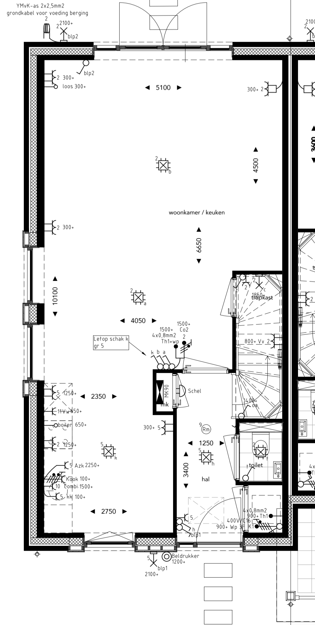
begane grond
