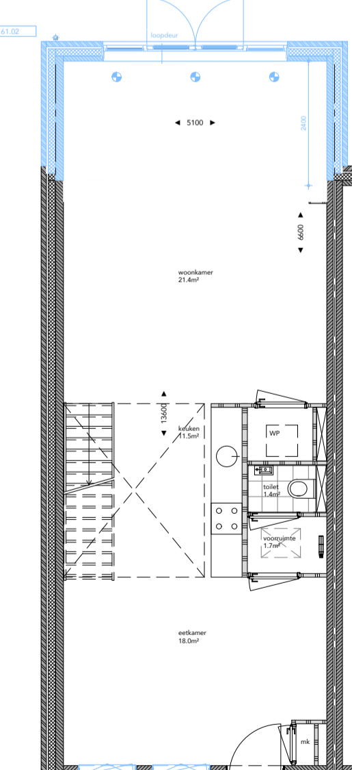
EERSTE VERDIEPING 61.02 2,4 mtr uitbouw achtergevel, opp uitbreiding: 10.8 m 2 go
