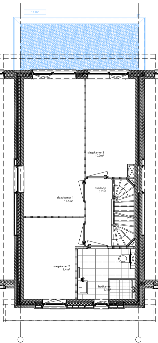
EERSTE VERDIEPING 11.02 2,4 mtr uitbouw achtergevel
