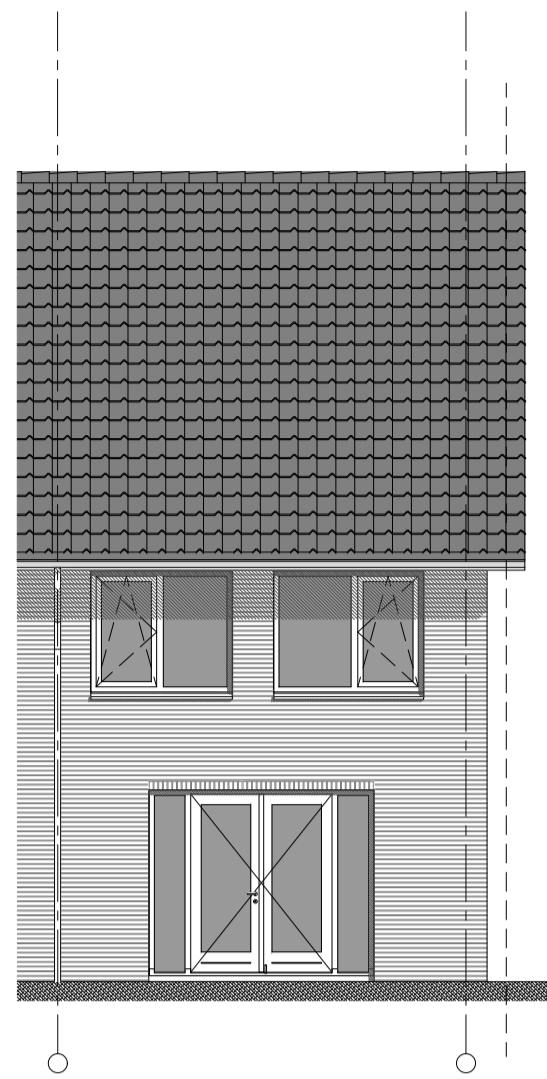
ACHTERGEVEL TYPE B-1 basis
