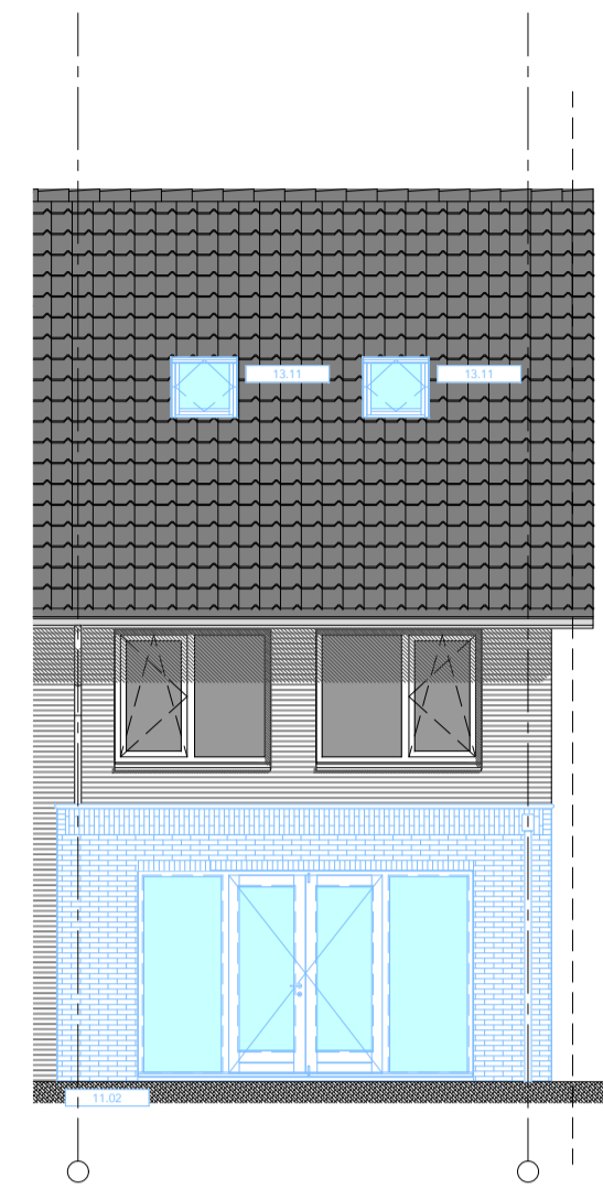
ACHTERGEVEL 11.02 2,4 mtr uitbouw achtergevel 13.11 dakraam type Velux GGL-MK04 ca.78x98cm
