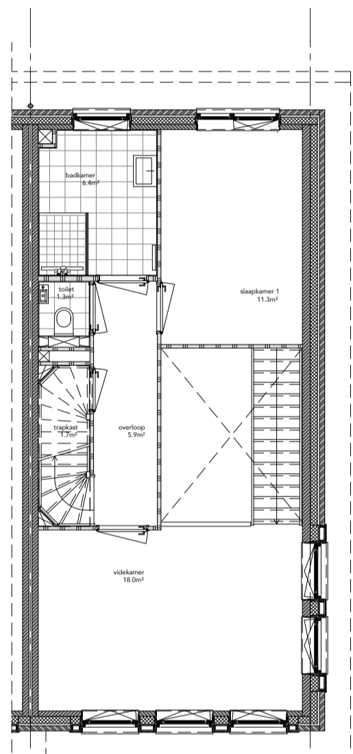
EERSTE VERDIEPING TYPE D-3b basis
