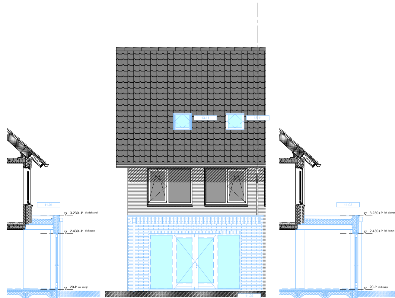
ACHTERGEVEL
