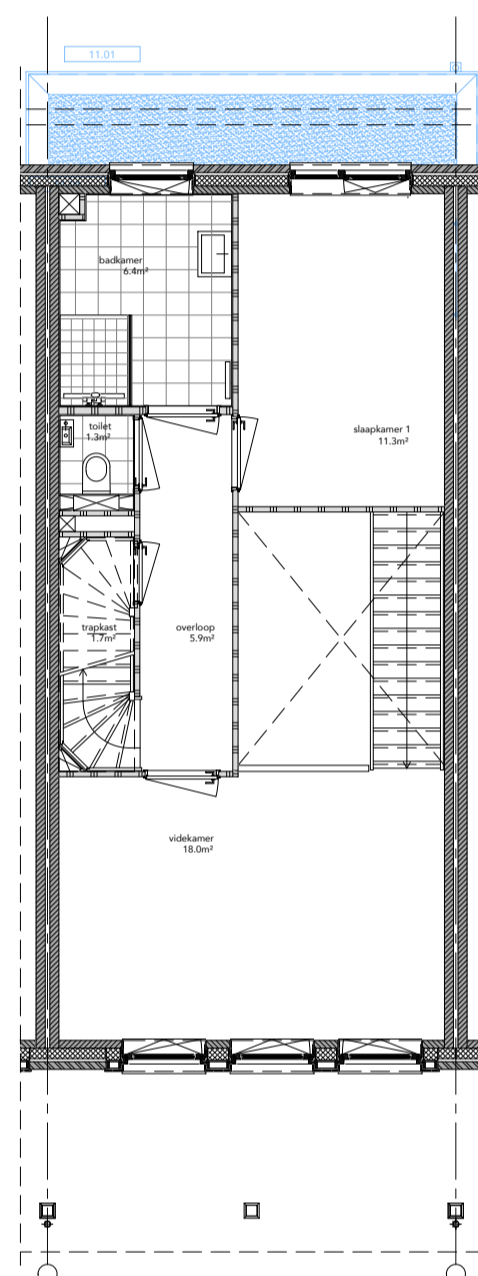
EERSTE VERDIEPING 61.01 1,2 mtr uitbouw achtergevel, opp uitbreiding: 5,4 m 2 go
