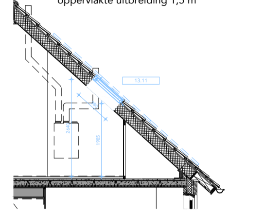
DOORSNEDE
