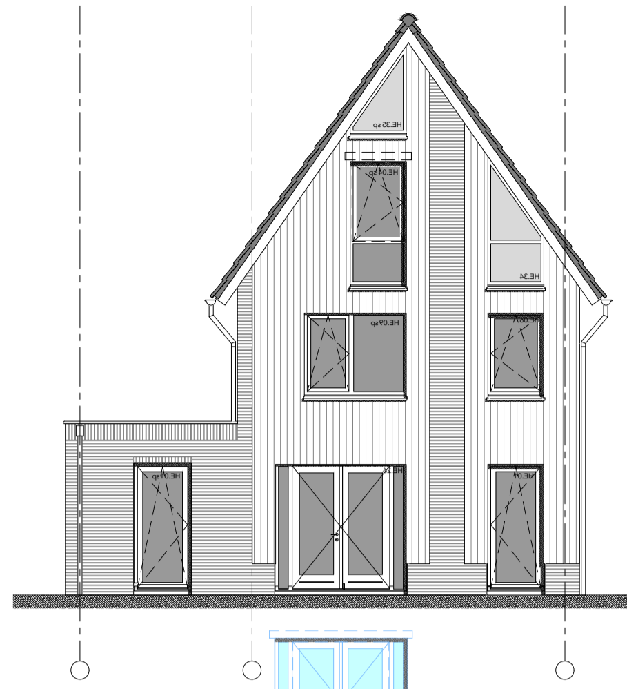
ACHTERGEVEL
