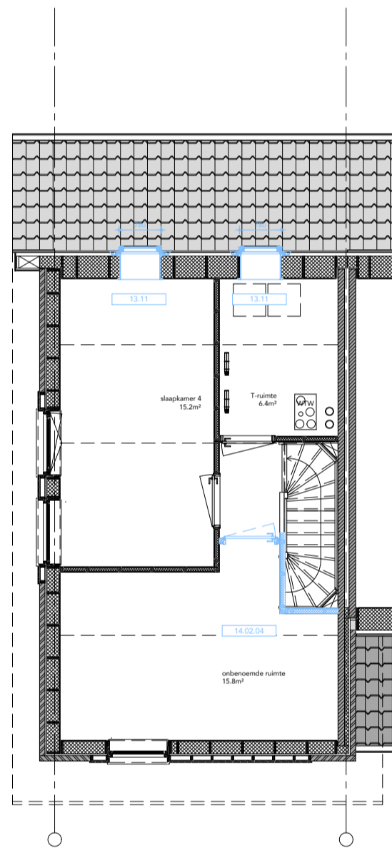
TWEDE VERDIEPING 13.11 dakraam type Velux GGL-MK04 ca.78x98cm 14.02.04 extra onbenoemde ruimte op zolderverdieping
