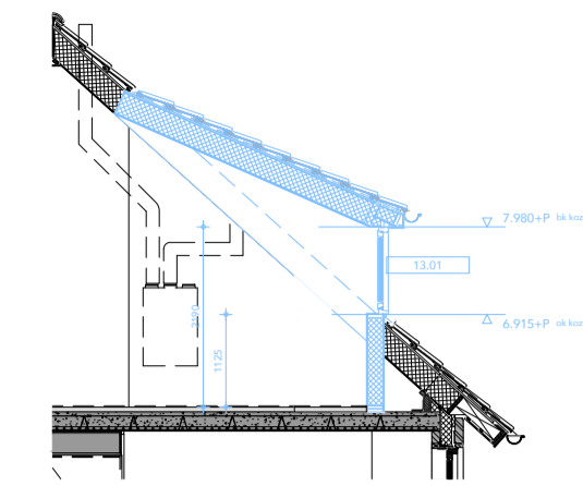
DOORSNEDE
