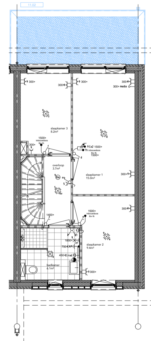
EERSTE VERDIEPING
