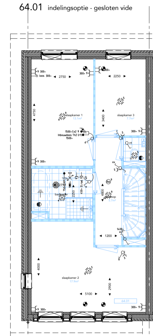
TWEDE VERDIEPING 64.01 indelingsoptie - gesloten vide
