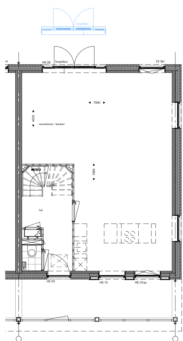
BEGANE GROND
