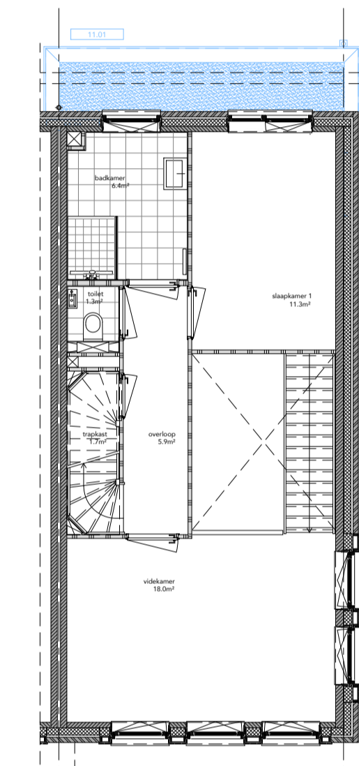
EERSTE VERDIEPING 61.01 1,2 mtr uitbouw achtergevel, opp uitbreiding: 5.4 m 2 go
