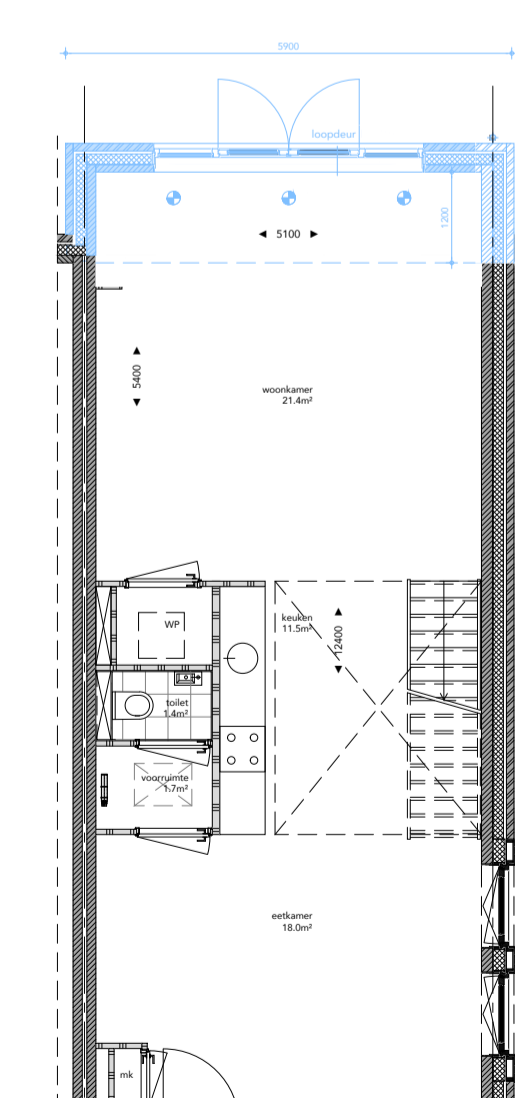
BEGANE GROND 61.01 1,2 mtr uitbouw achtergevel opp uitbreiding: 5.4 m 2 go
