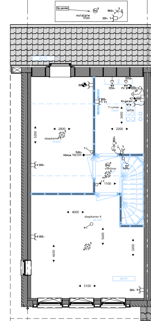
TWEDE VERDIEPING 64.01 indelingsoptie - gesloten vide
