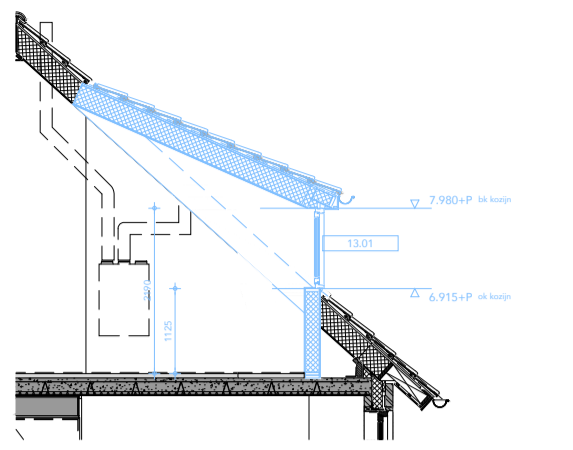
DOORSNEDE 13.01 dakkapel, breedte +/- 1,94 mtr (binnenmaat)
