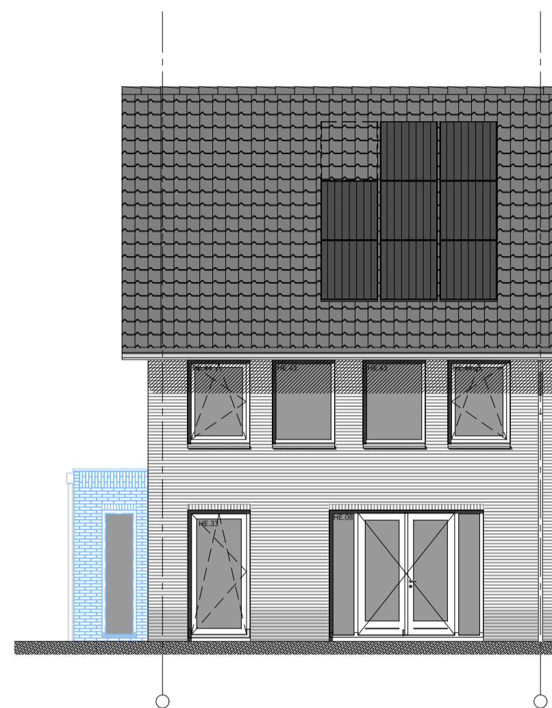
ACHTERGEVEL
