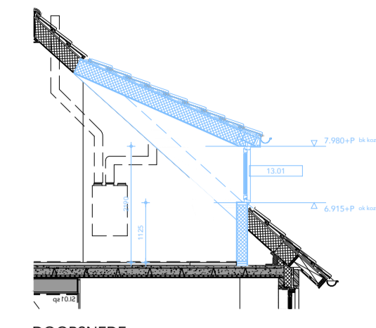
DOORSNEDE 73.01 dakkapel, breedte +/- 1,9 mtr (binnenmaat)
