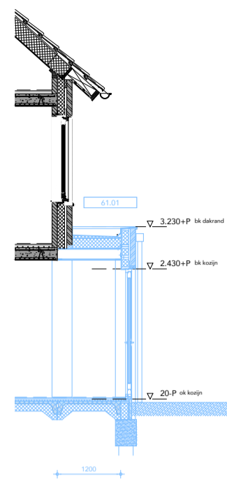
ACHTERGEVEL 61.01 1,2 mtr uitbouw achtergevel, opp uitbreiding: 5,4 m 2 go
