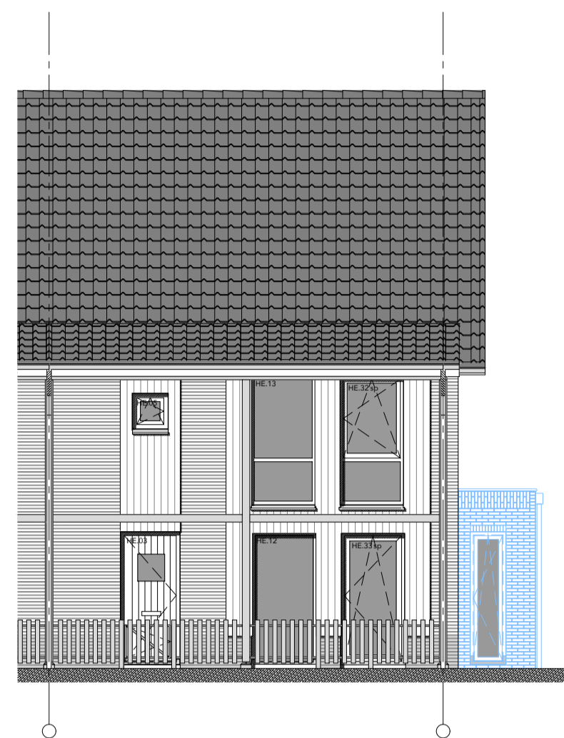
VOORGEVEL
