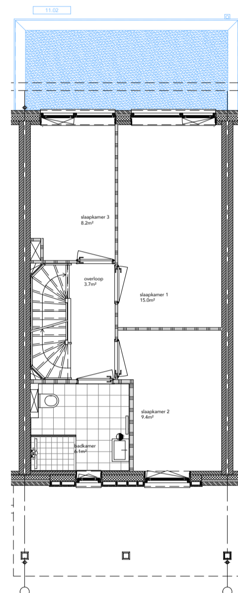
EERSTE VERDIEPING
