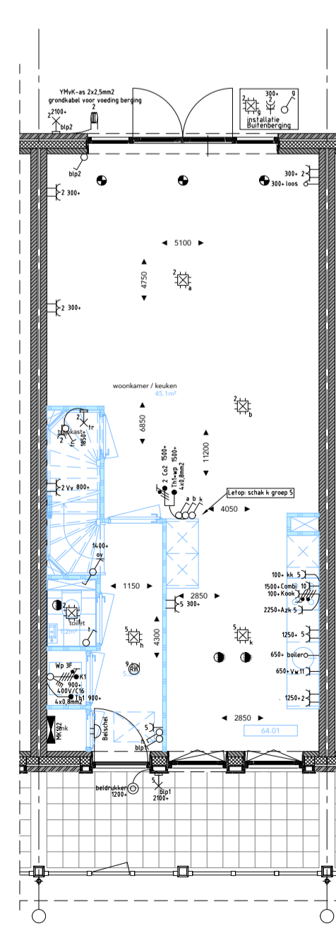
BEGANE GROND 64.01 indelingsoptie – gesloten vide
