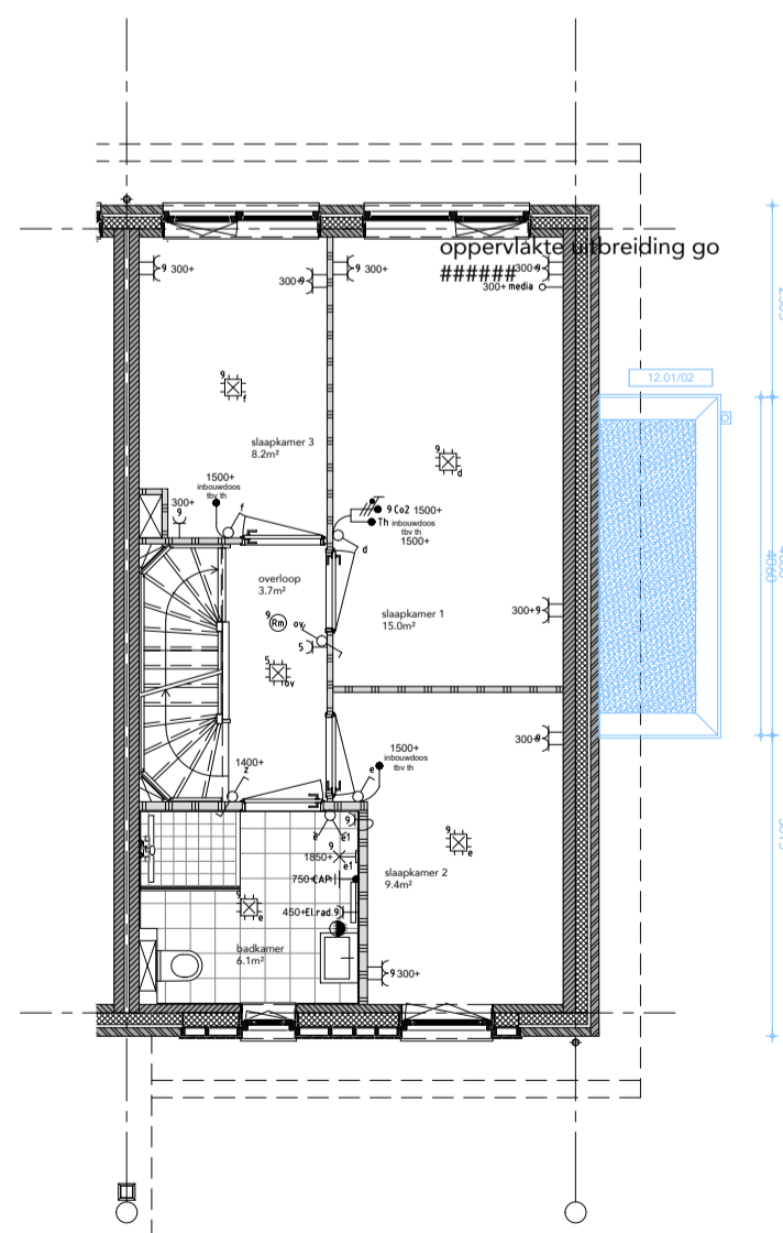
EERSTE VERDIEPING
