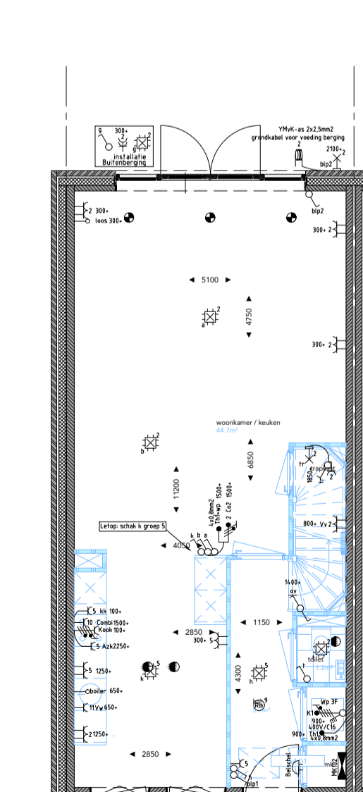
EERSTE VERDIEPING 64.01 indelingsoptie - gesloten vide
