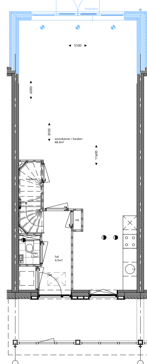
BEGANE GROND
