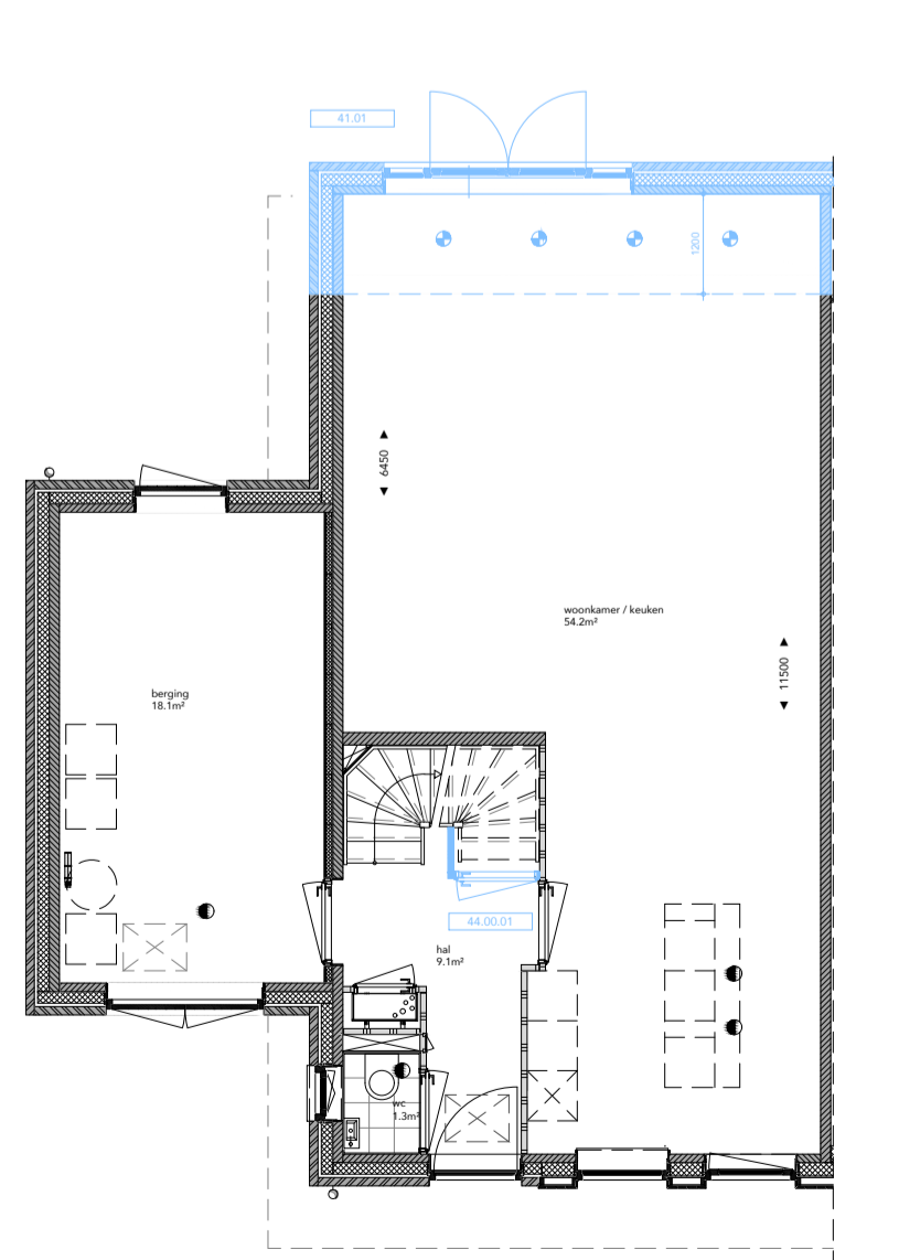
BEGANE GROND
