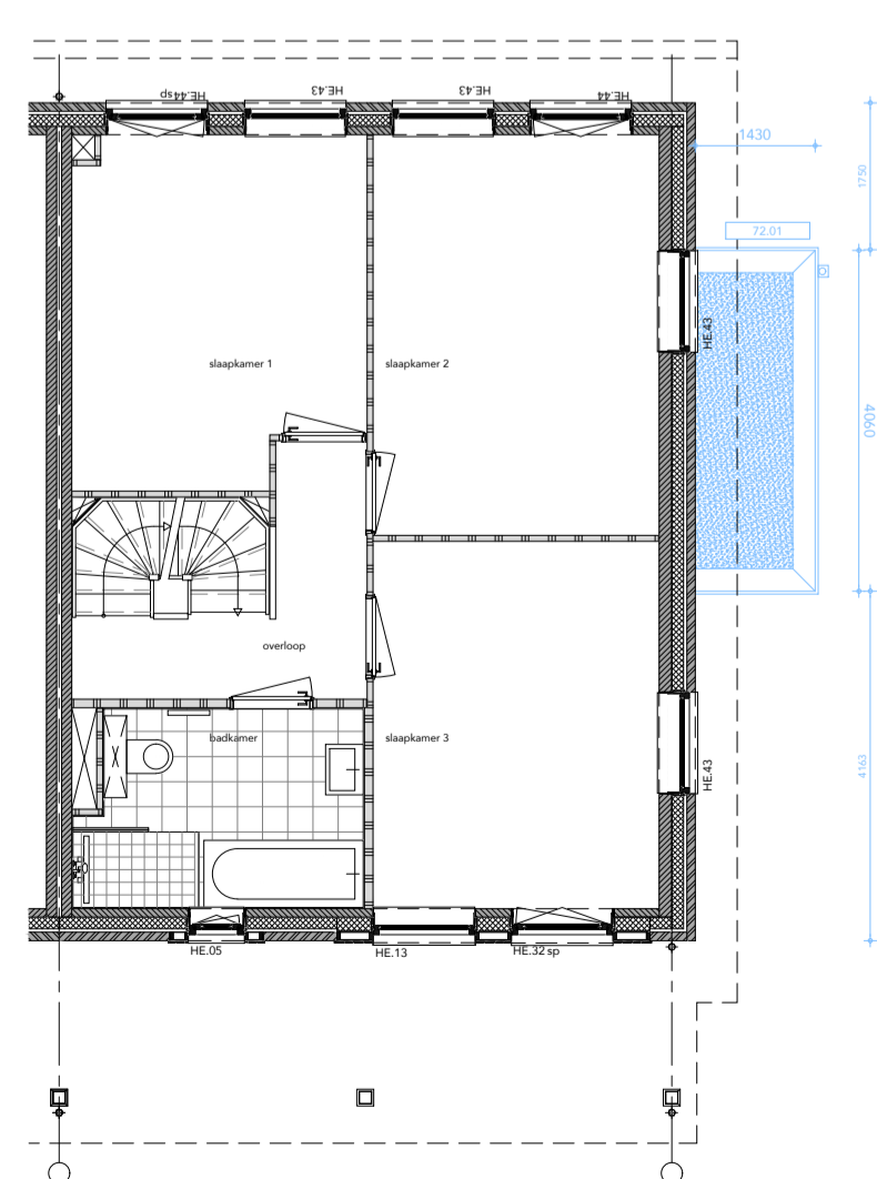
EERSTE VERDIEPING
