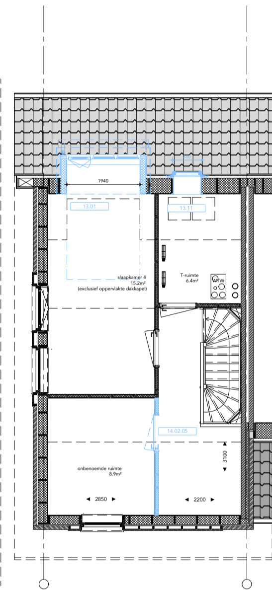
TWEDE VERDIEPING 13.01 dakkapel, breedte +/- 1,94 mtr (binnenmaat) oppervlakte uitbreiding 1,5 m² 13.11 dakraam type Velux GGL-MK04 ca.78x98cm 14.02.05 extra onbenoemde ruimte op zolderverdieping
