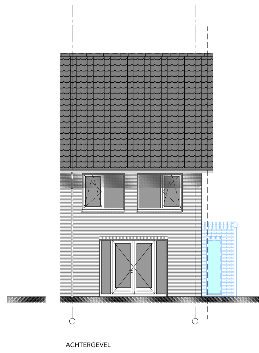
ACHTERGEVEL
