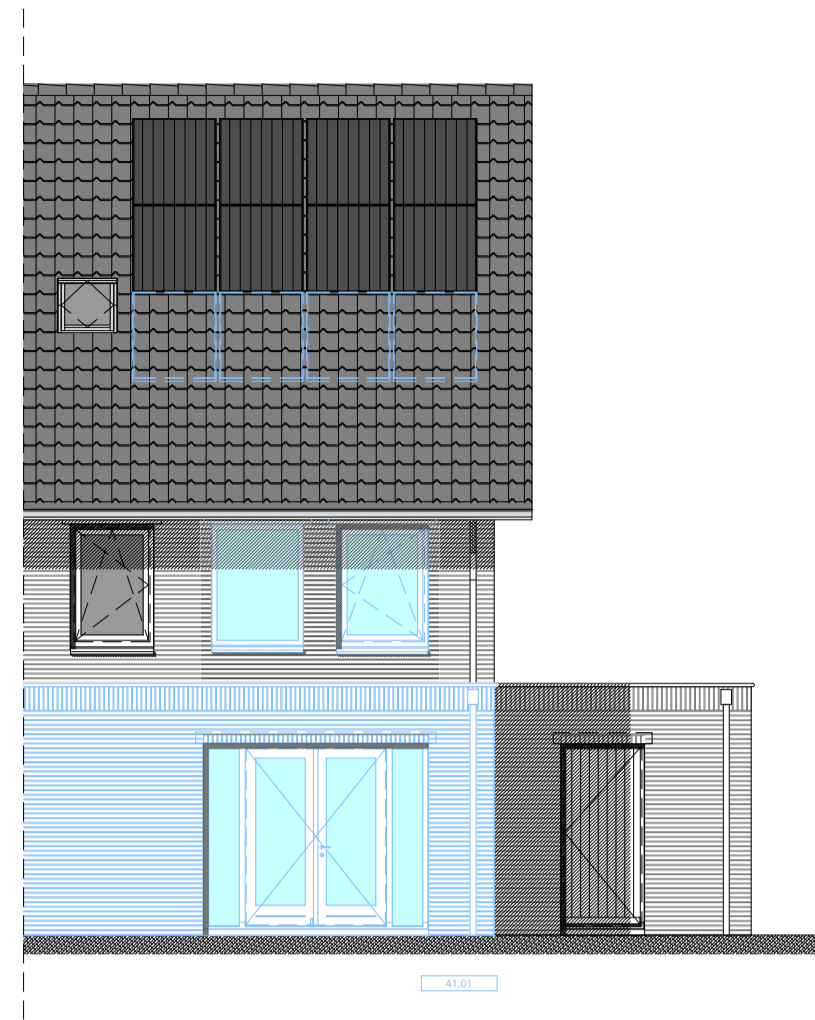
ACHTERGEVEL
