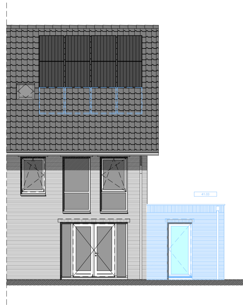
ACHTERGEVEL
