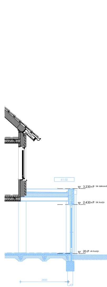
ACHTERGEVEL 61.02 2,4 mtr uitbouw achtergevel, opp uitbreiding: 10.8 m 2 go
