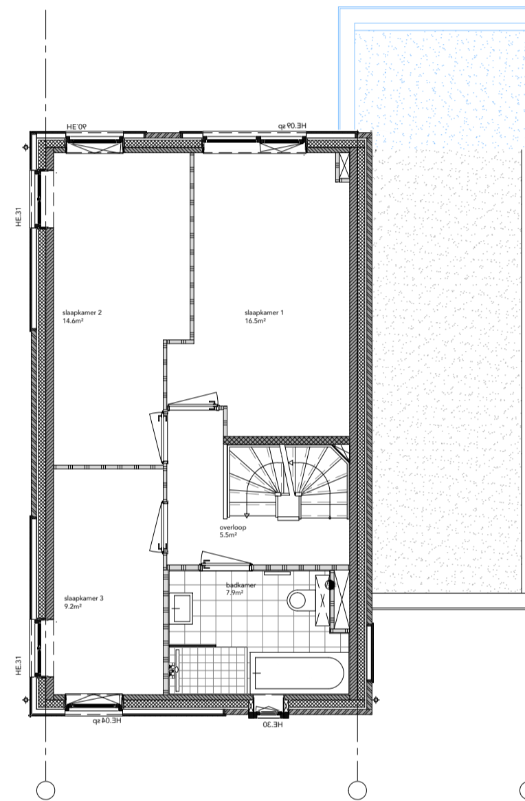
EERSTE VERDIEPING
