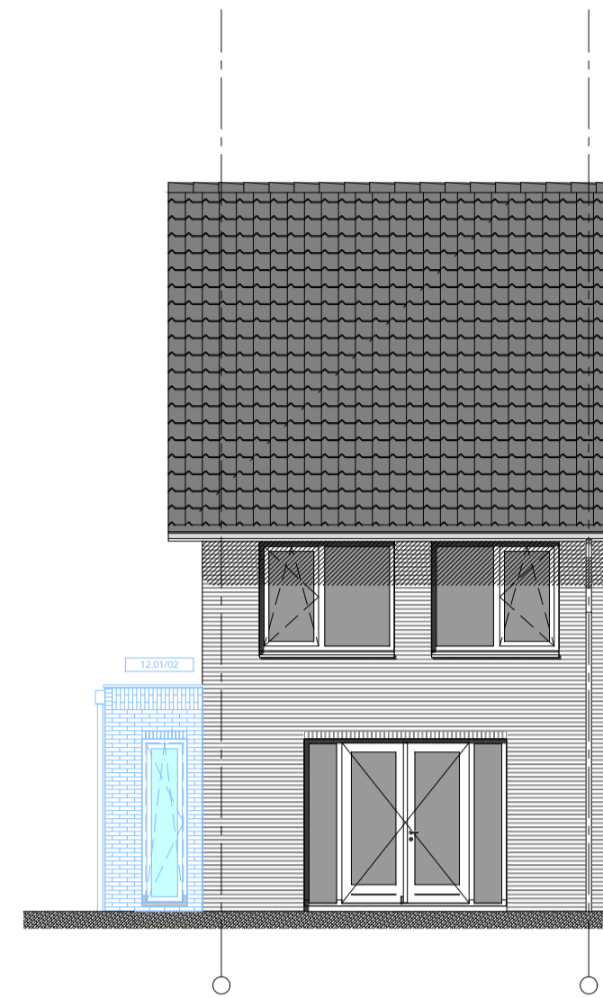
ACHTERGEVEL
