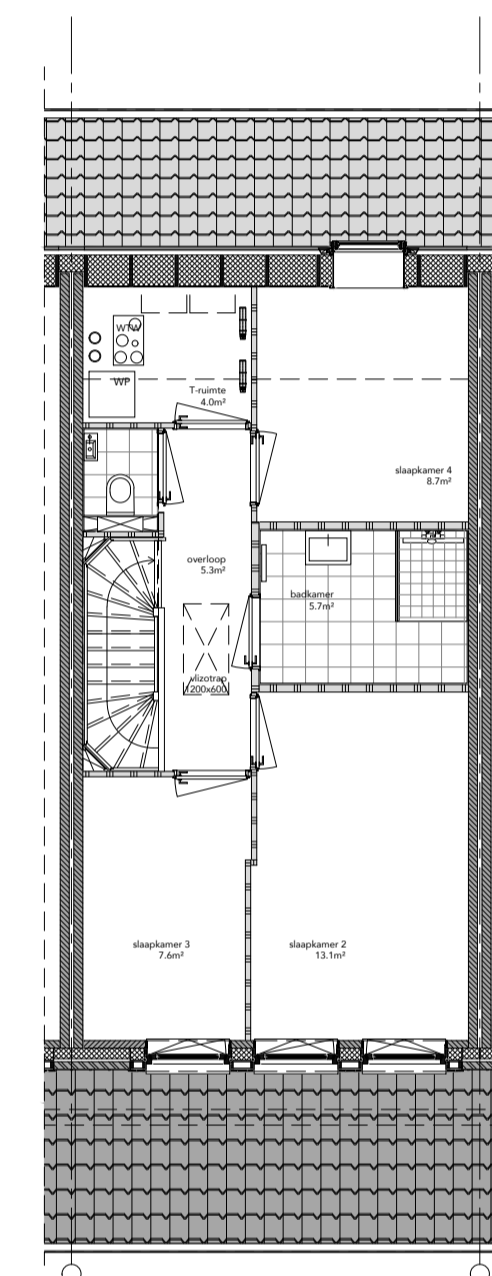
TWEDE VERDIEPING TYPE D-1b basis
