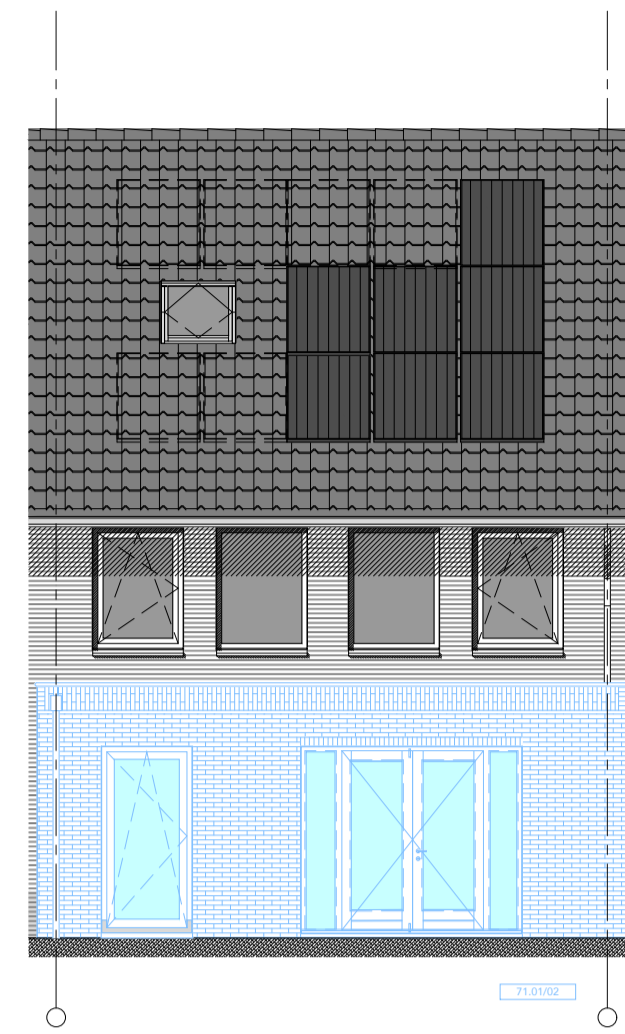
ACHTERGEVEL
