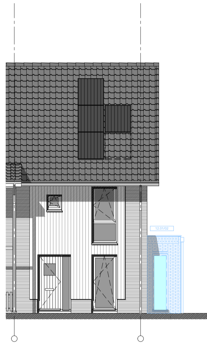
VOORGEVEL
