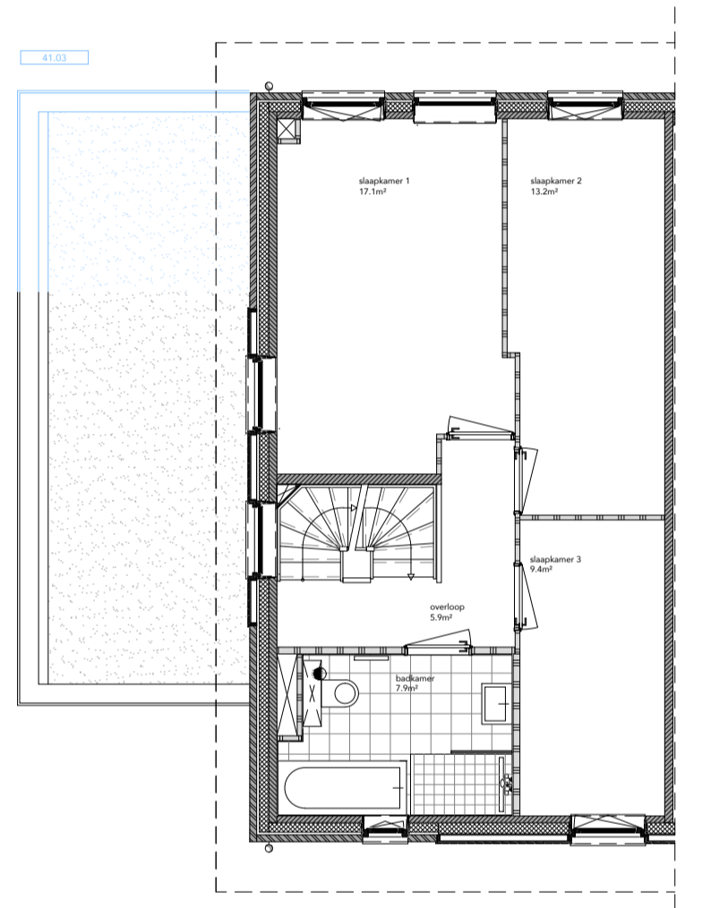
EERSTE VERDIEPING
