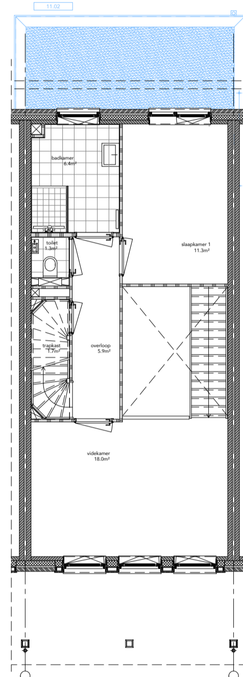
EERSTE VERDIEPING 61.02 2,4 mtr uitbouw achtergevel, opp uitbreiding: 10,8 m 2 go
