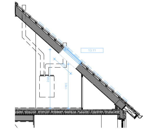
DOORSNEDE 13.11 dakraam type Velux GGL-MK04 ca.78x98cm
