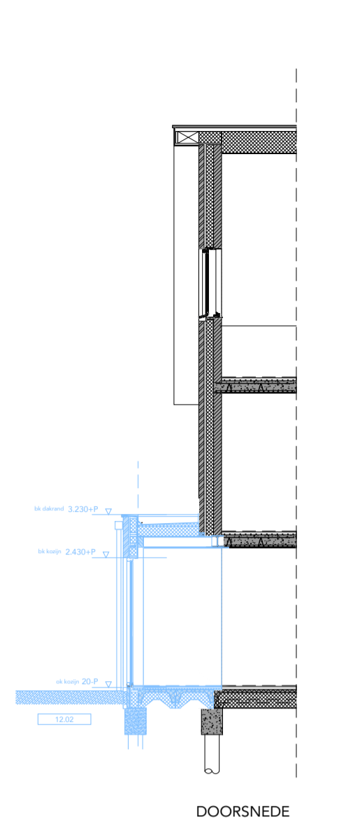
DOORSNEDE
