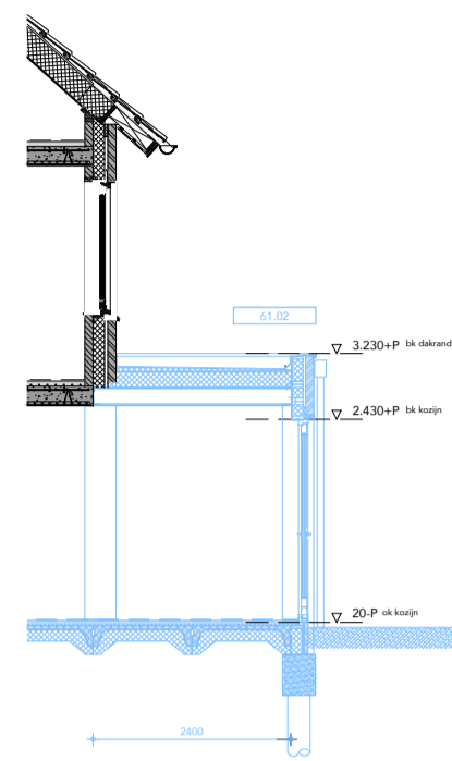
ACHTERGEVEL 61.02 2,4 mtr uitbouw achtergevel, opp uitbreiding: 10,8 m 2 go
