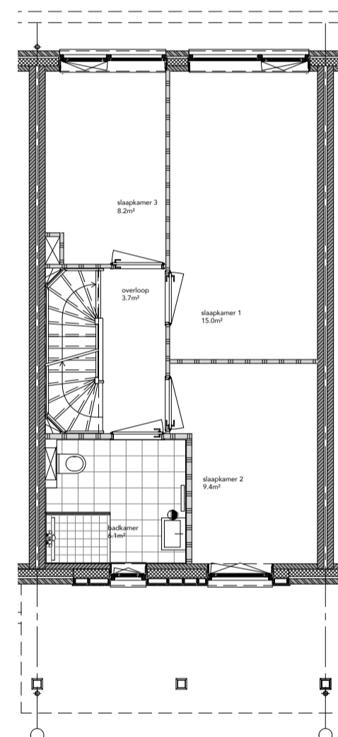
EERSTE VERDIEPING
