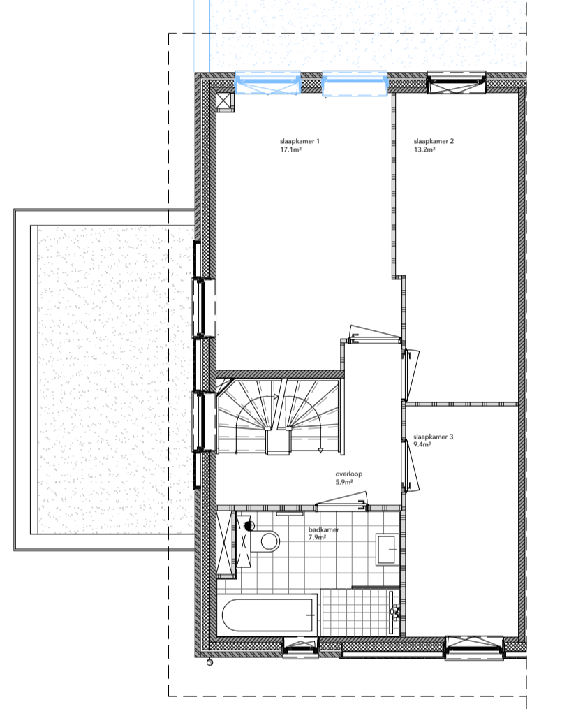
EERSTE VERDIEPING
