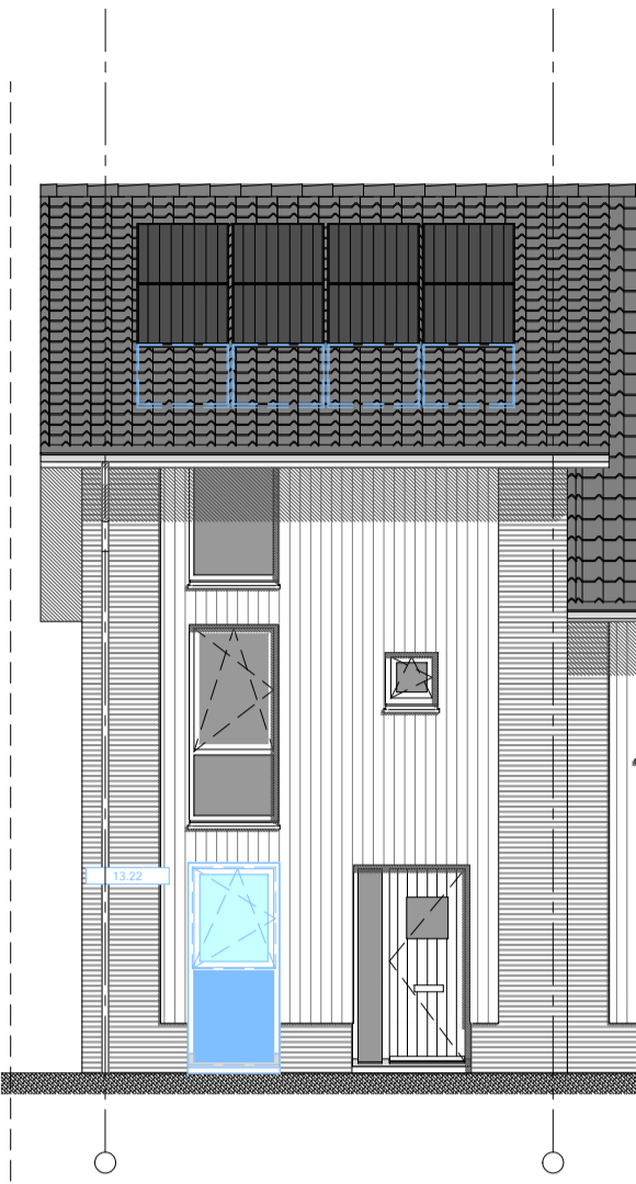
VOORGEVEL 13.22 dichtzetten glasvlak laag kozijn voorgevel met colorbel paneel. kleur: idem voordeur
