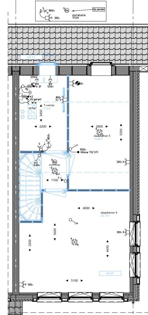
TWEDE VERDIEPING 64.01 indelingsoptie - gesloten vide 63.11 dakraam type Velux GGL-MK04 ca.78x98cm
