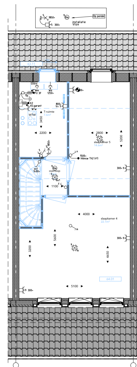
TWEDE VERDIEPING 64.01 indelingsoptie – gesloten vide 63.11 dakraam type Velux GGL-MK04 ca.78x98cm
