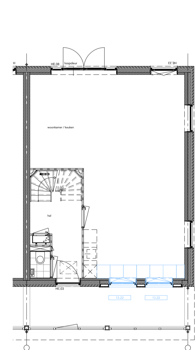
BEGANE GROND
