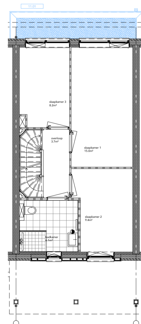
EERSTE VERDIEPING
