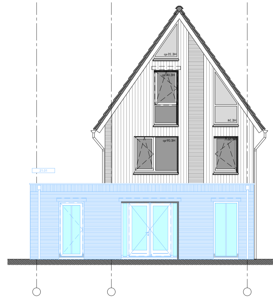
ACHTERGEVEL
