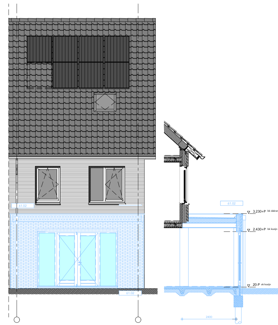
ACHTERGEVEL 61.02 2,4 mtr uitbouw achtergevel, opp uitbreiding: 10.8 m 2 go
