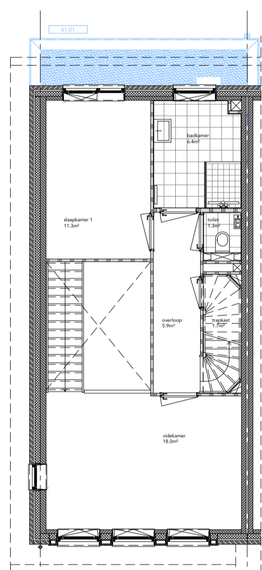
ACHTERGEVEL 61.01 1,2 mtr uitbouw achtergevel, opp uitbreiding: 5.4 m 2 go
