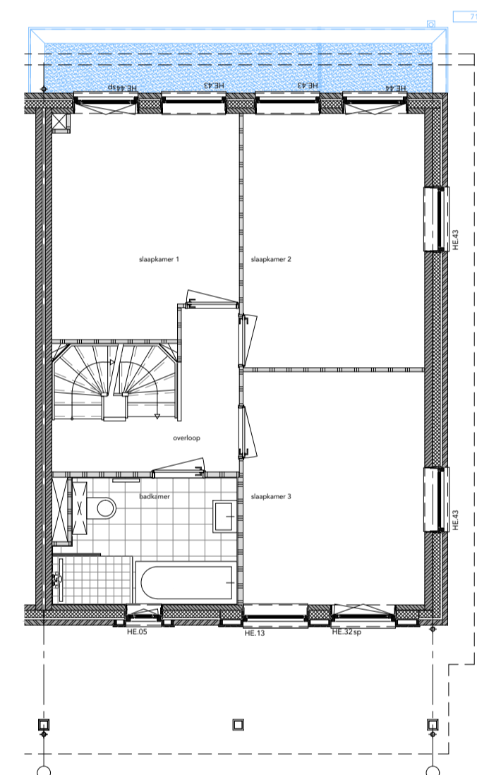
EERSTE VERDIEPING
