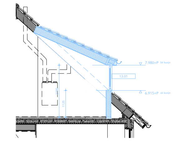
DOORSNEDE 13.01 dakkapel, breedte +/- 1,94 mtr (binnenmaat) oppervlakte uitbreiding 1,5 m²
