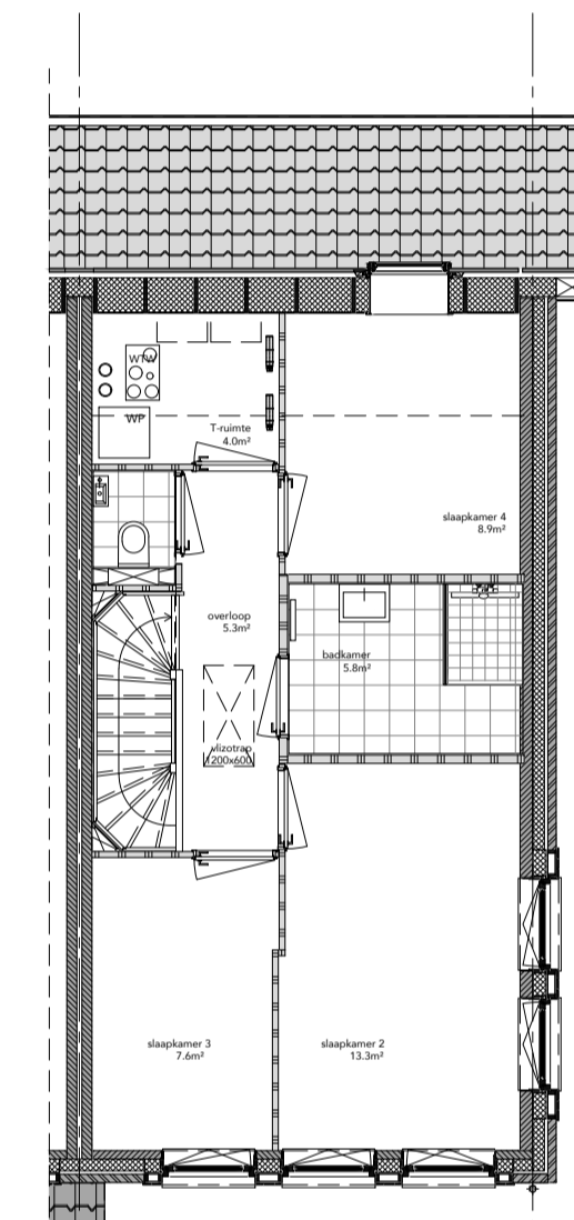
TWEDE VERDIEPING TYPE D-3b basis
