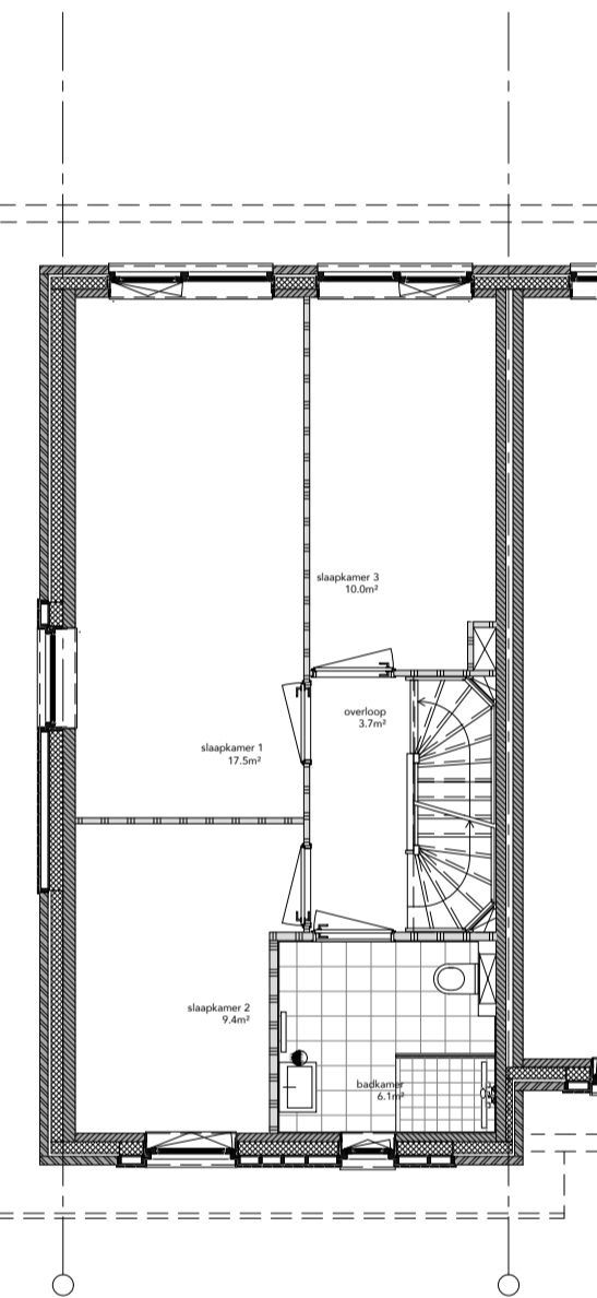
EERSTE VERDIEPING TYPE B-1 basis
