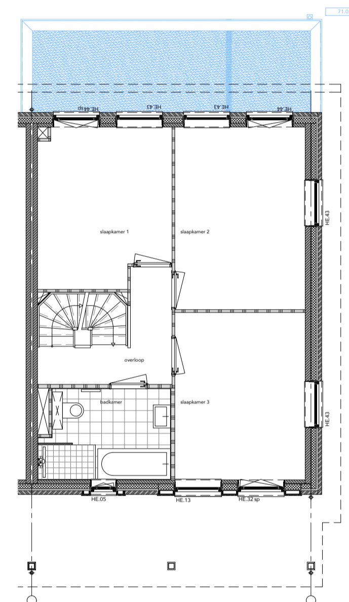
EERSTE VERDIEPING
