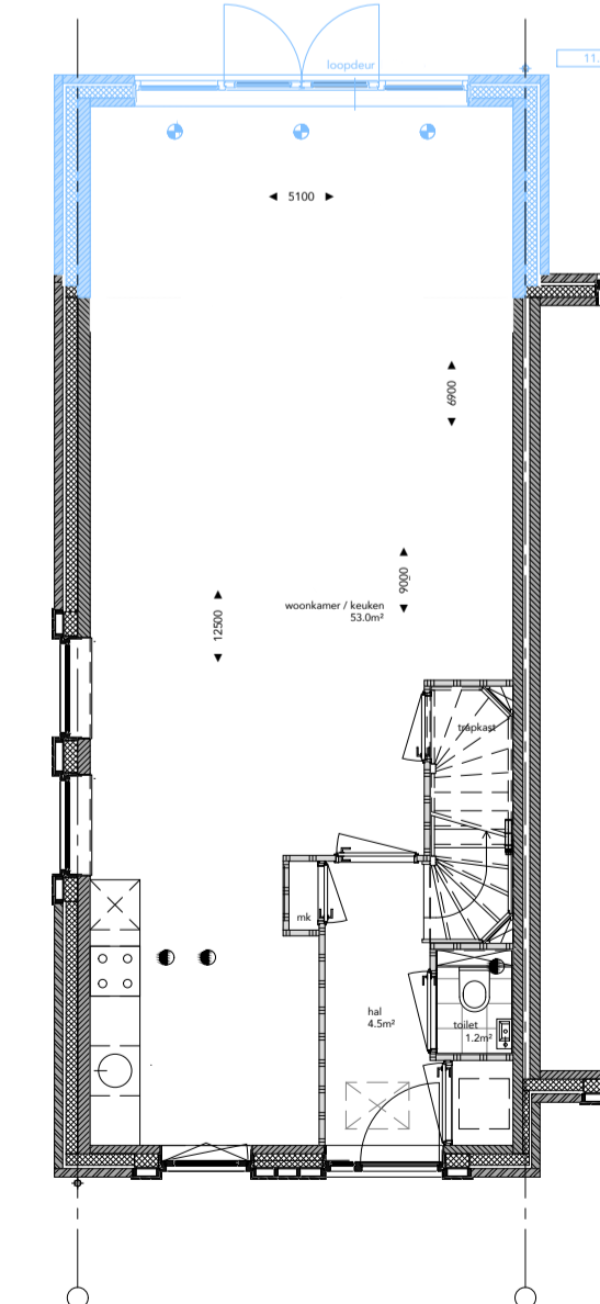
BEGANE GROND 11.02 2,4 mtr uitbouw achtergevel oppervlakte uitbreiding go 12,2m²
