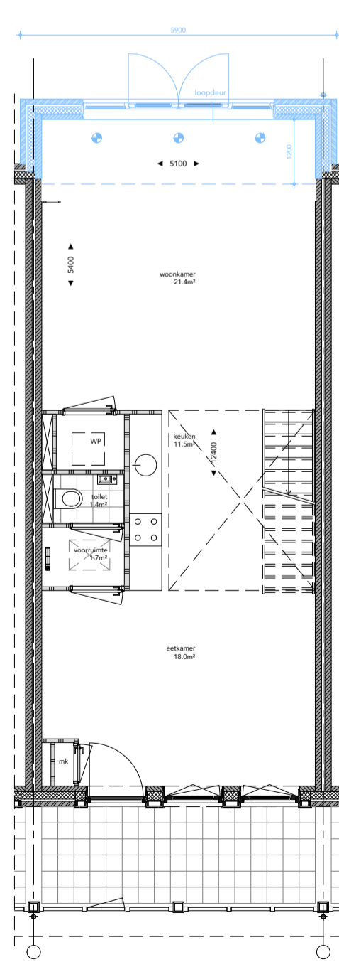
BEGANE GROND 61.01 1,2 mtr uitbouw achtergevel opp uitbreiding: 5,4 m 2 go
