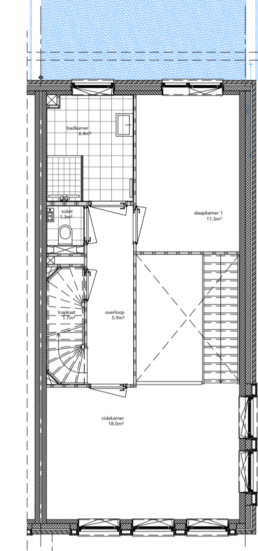
EERSTE VERDIEPING 61.02 2,4 mtr uitbouw achtergevel, opp uitbreiding: 10.8 m 2 go
