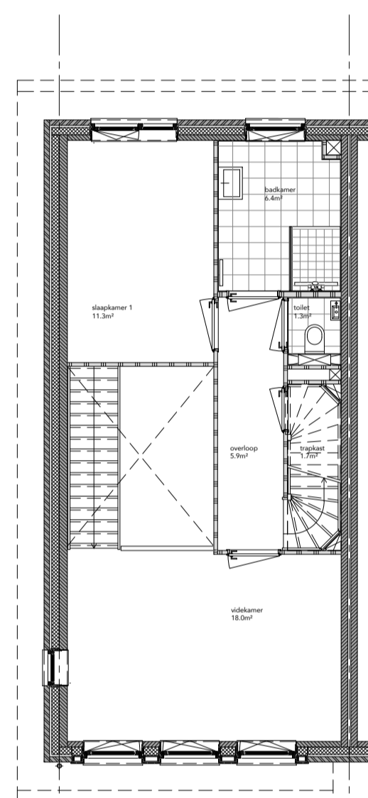
EERSTE VERDIEPING TYPE D-2b basis
