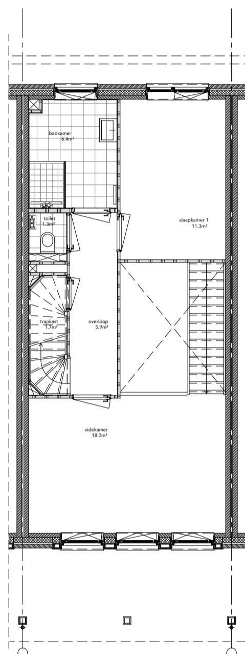
EERSTE VERDIEPING TYPE D-1b basis
