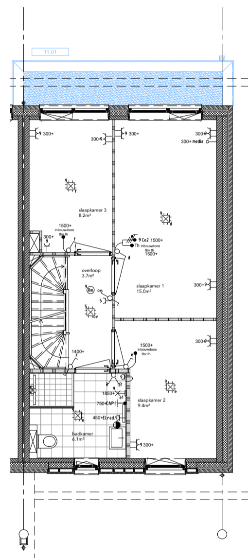
EERSTE VERDIEPING
