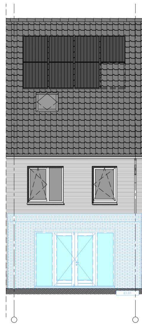
ACHTERGEVEL 61.01 1,2 mtr uitbouw achtergevel, opp uitbreiding: 5,4 m 2 go
