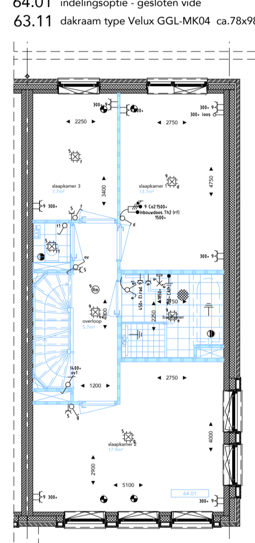
EERSTE VERDIEPING 64.01 indelingsoptie - gesloten vide
