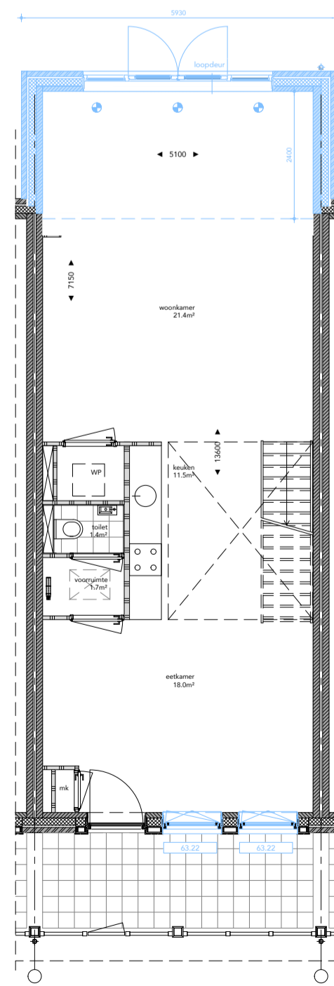
BEGANE GROND 61.02 2,4 mtr uitbouw achtergevel, opp uitbreiding: 10,8 m 2 go 63.22 dichtzetten glasvlak met colorbel paneel
