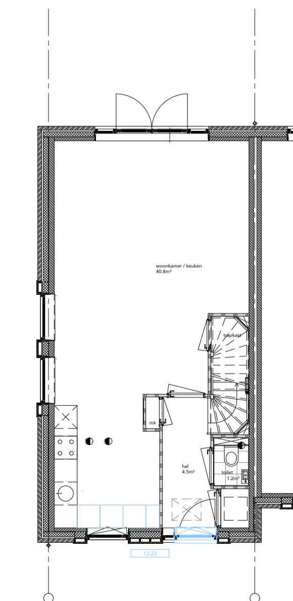
BEGANE GROND 13.22 dichtzetten glasvlak laag kozijn voorgevel met colorbel paneel. kleur: idem voordeur
