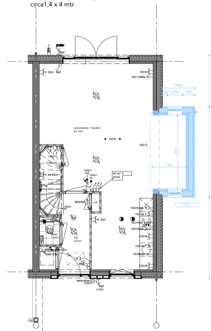
BEGANE GROND
