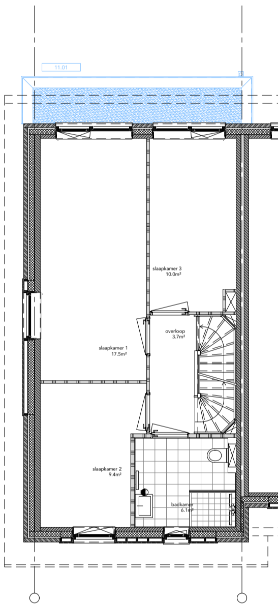
EERSTE VERDIEPING 11.01 1,2 mtr uitbouw achtergevel
