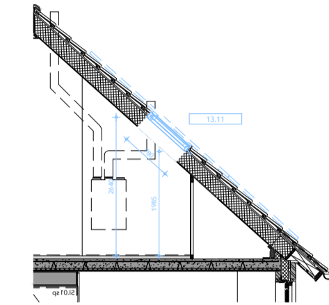
DOORSNEDE 73.11 dakraam type Velux GGL-MK04 ca.78x98cm
