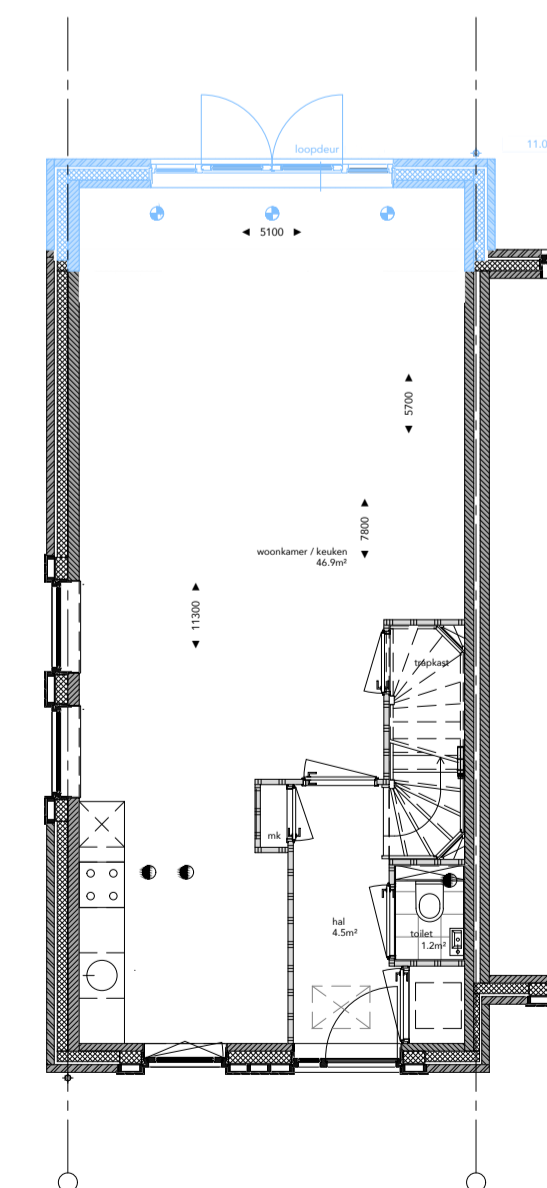
BEGANE GROND 11.01 1,2 mtr uitbouw achtergevel oppervlakte uitbreiding go 6,1m²
