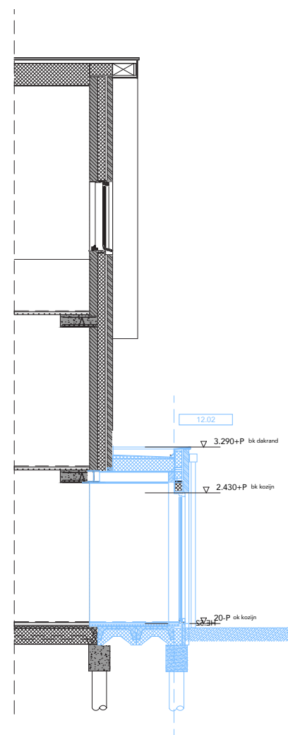
DOORSNEDE
