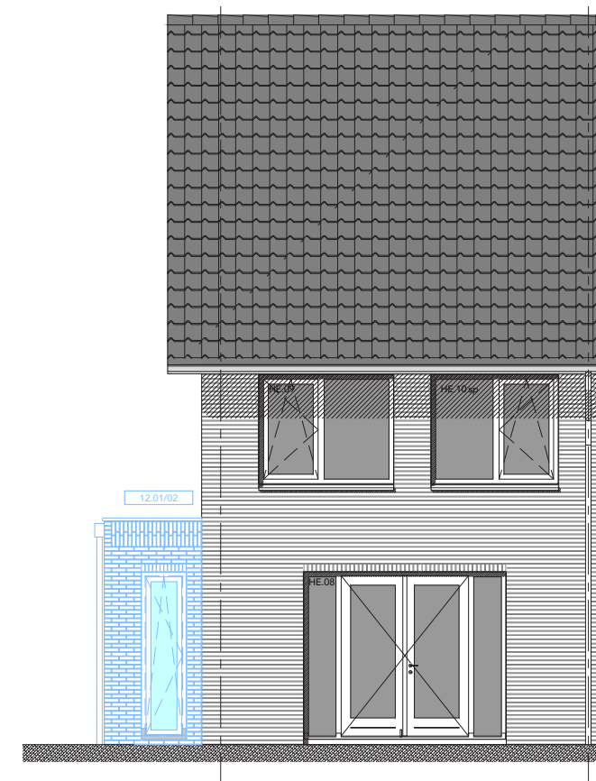
ACHTERGEVEL
