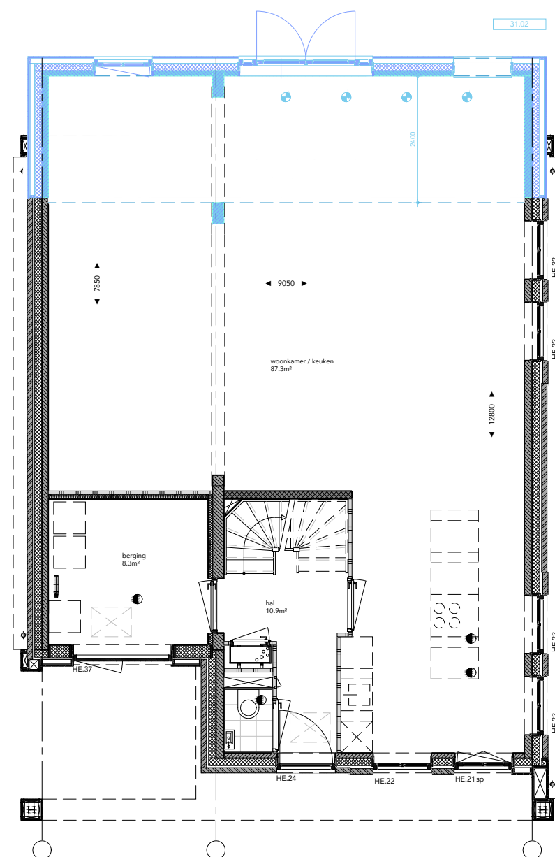
BEGANE GROND
