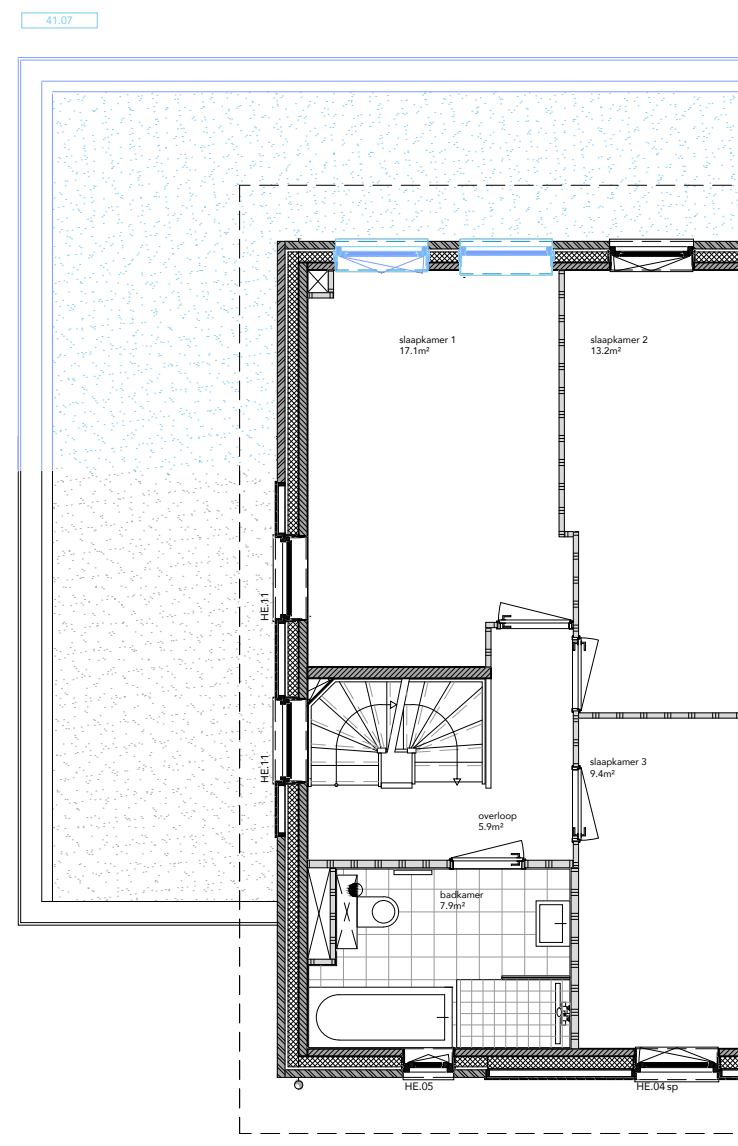
EERSTE VERDIEPING
