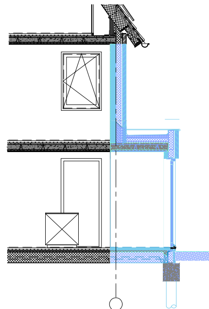
DOORSNEDE
