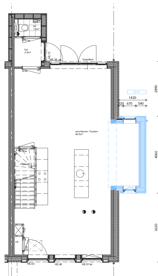
BEGANE GROND
