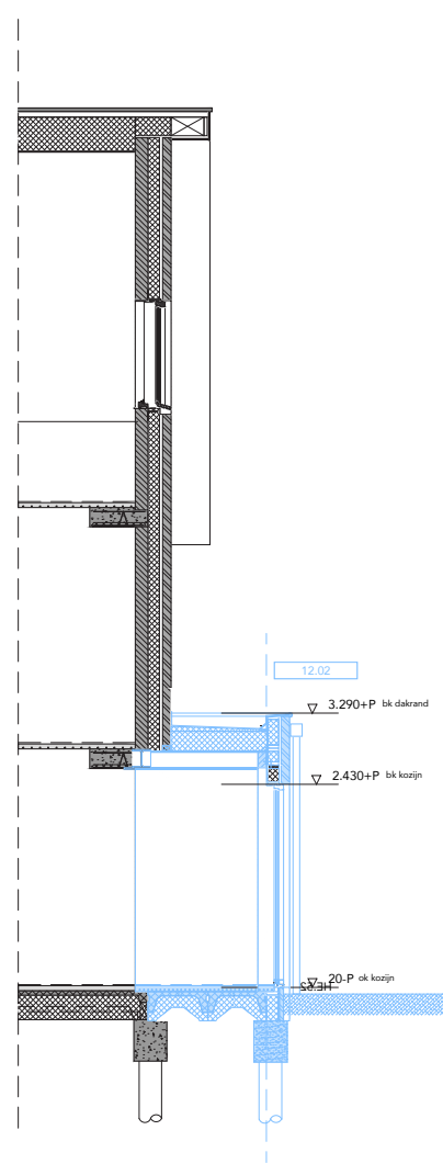
VOORGEVEL
