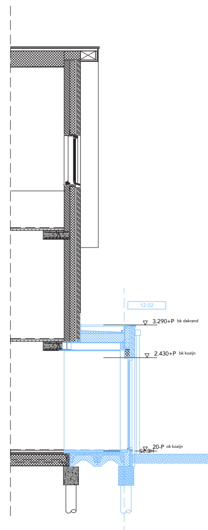
DOORSNEDE
