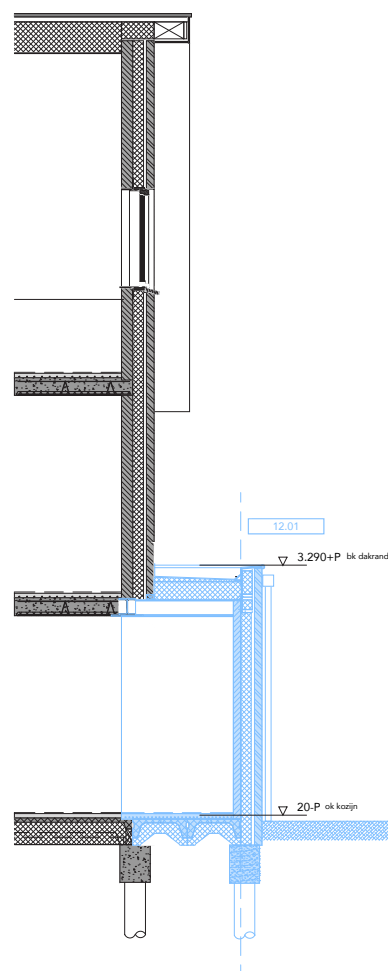
DOORSNEDE
