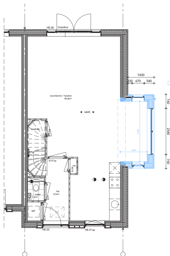
BEGANE GROND
