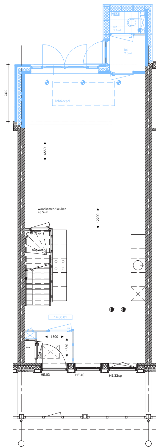
BEGANE GROND
