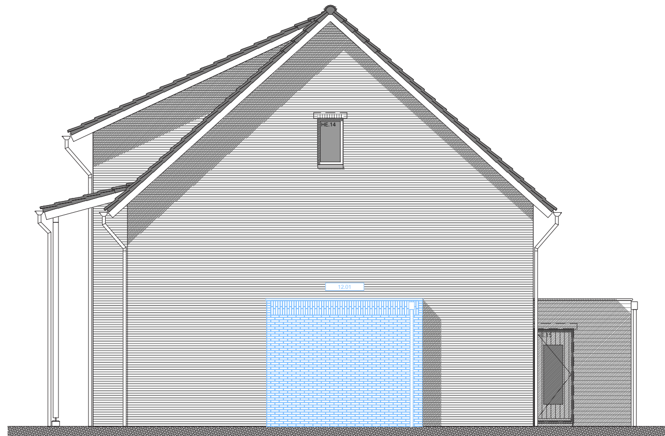
ZIJGEVEL
