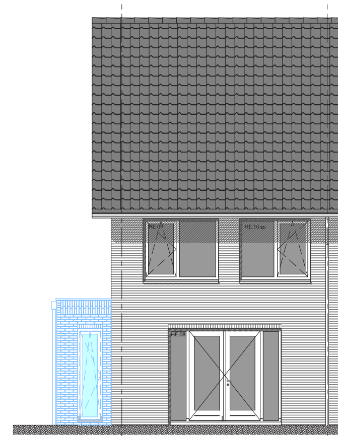
ACHTERGEVEL
