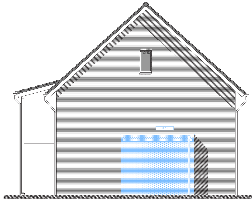
ZIJGEVEL
