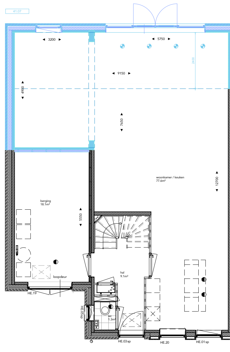
BEGANE GROND
