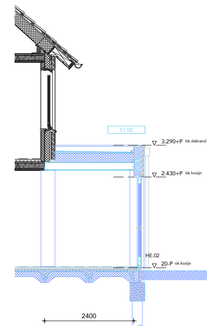
DOORSNEDE
